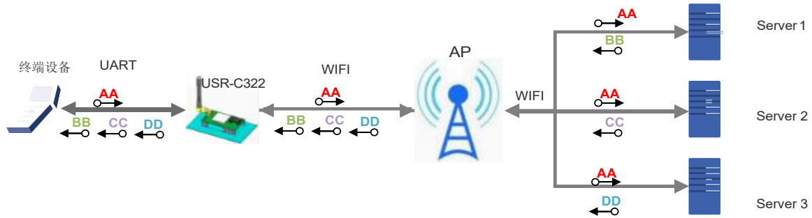
图 9 TCP Server
