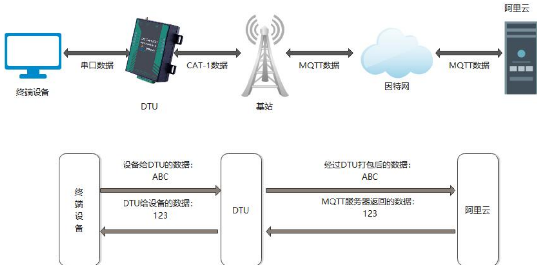
图 1 通信拓扑图
