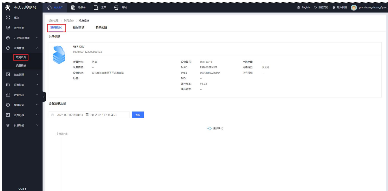
图 72 设备概况
