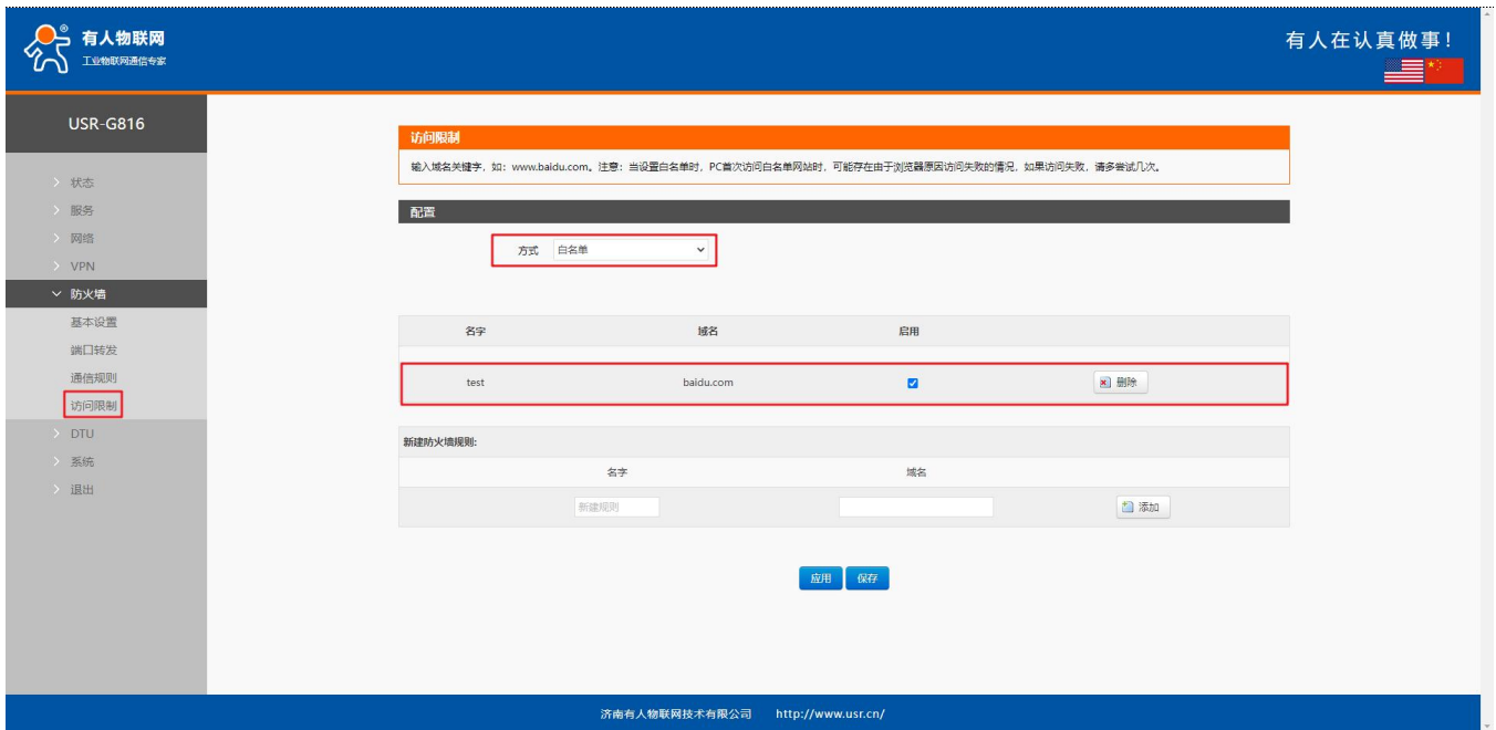
图 64 域名白名单
