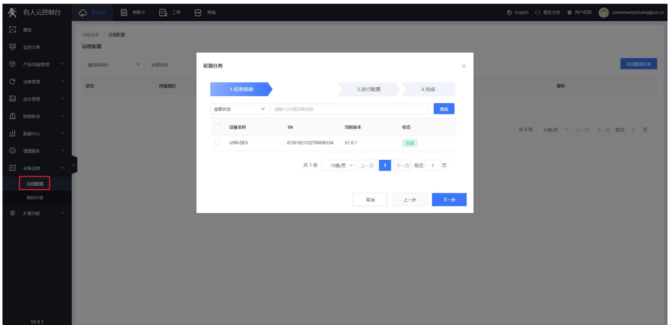
图 78 远程配置（二）
