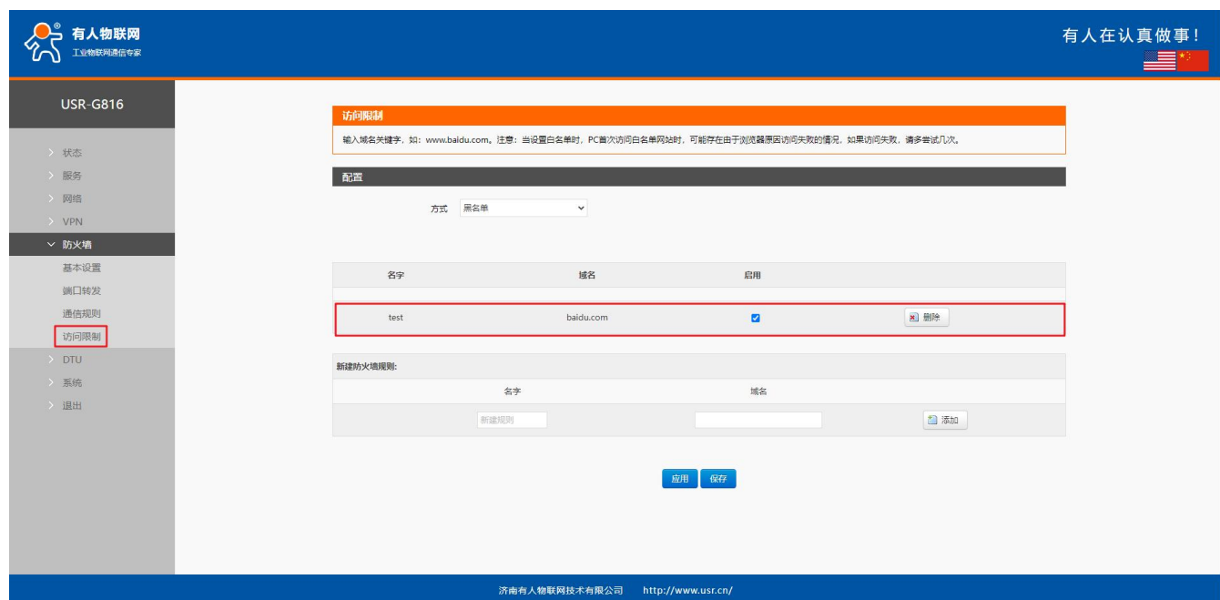
图 63 域名黑名单
