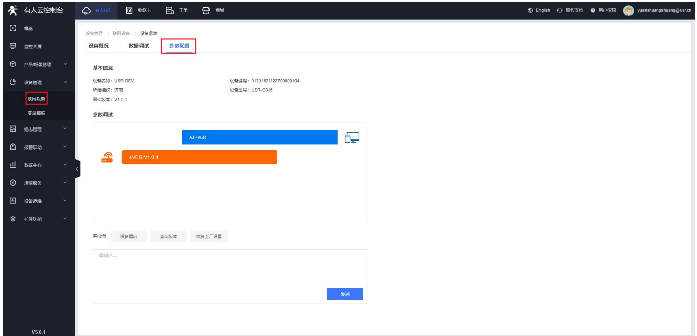
图 74 参数配置
