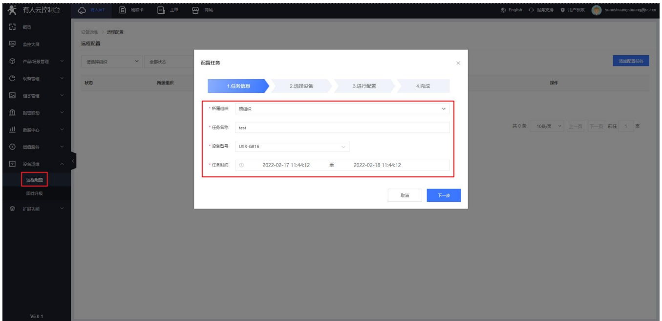
图 77 远程配置（一）
