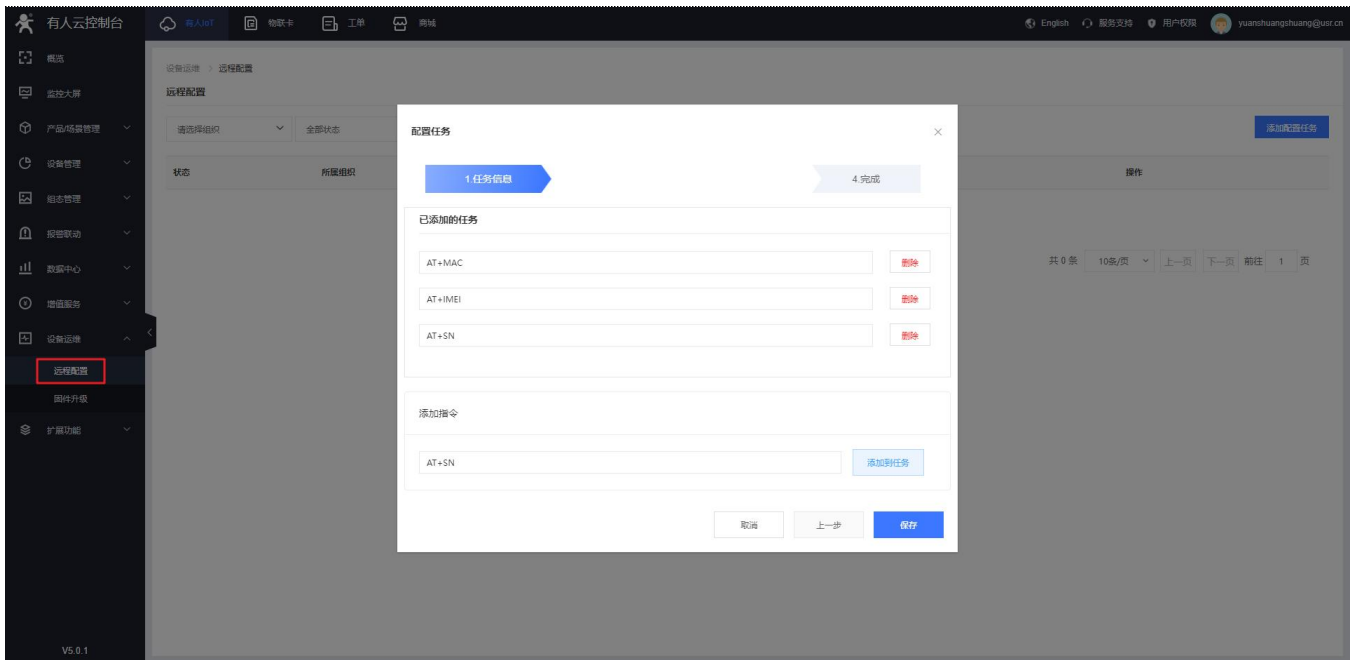
图 79 远程配置（三）
