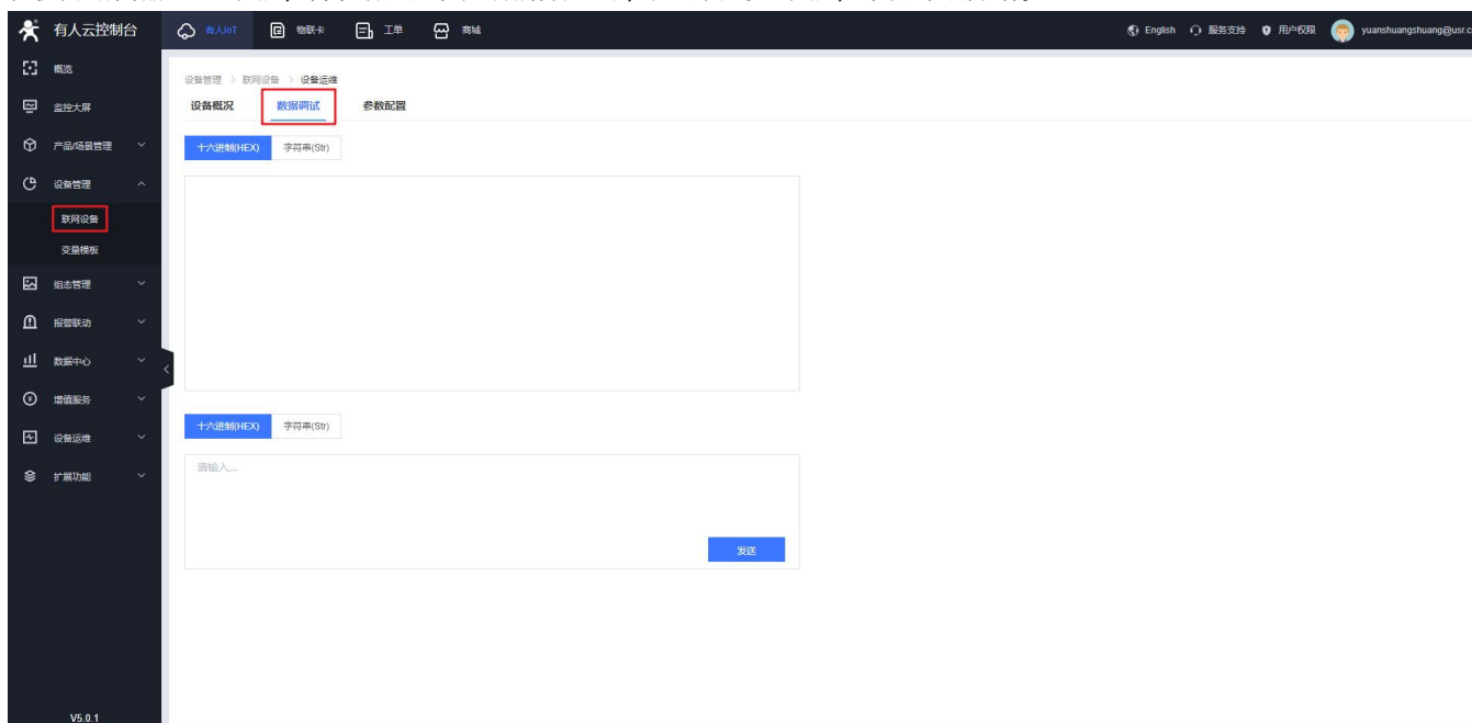
图 73 数据调试
