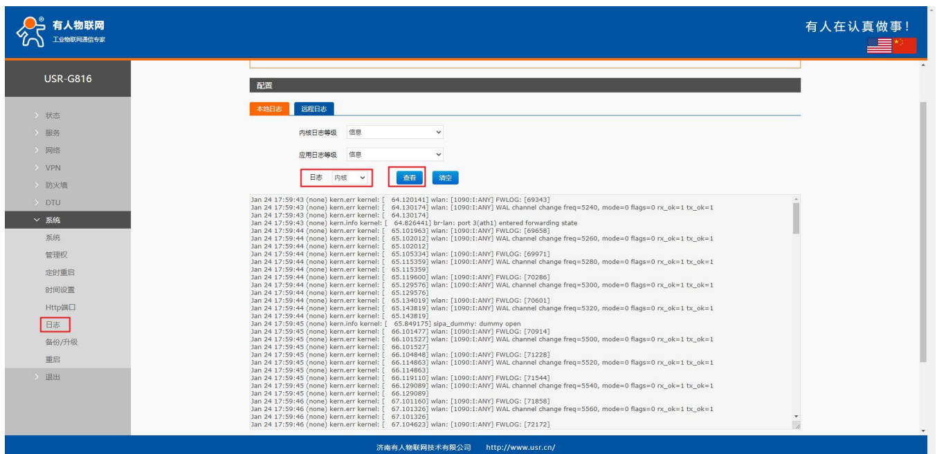
图 16 内核 log
