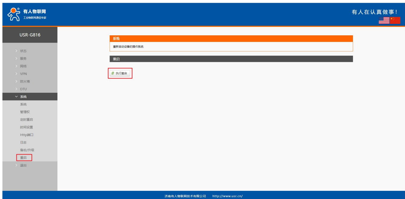
图 13 重启页面
