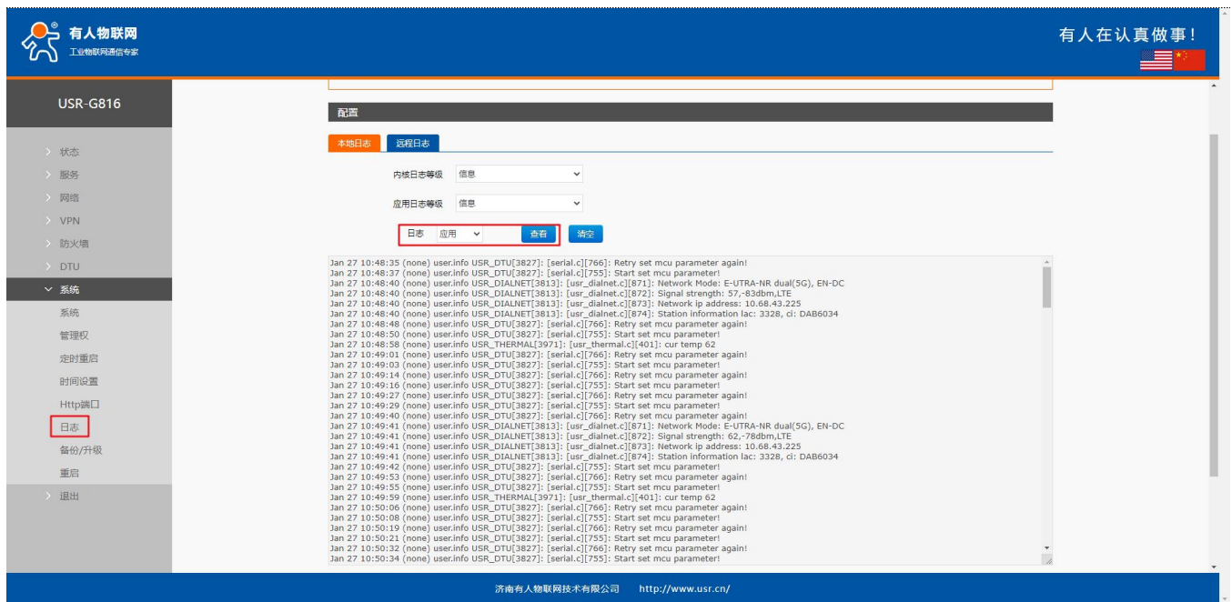
图 17 应用 log
