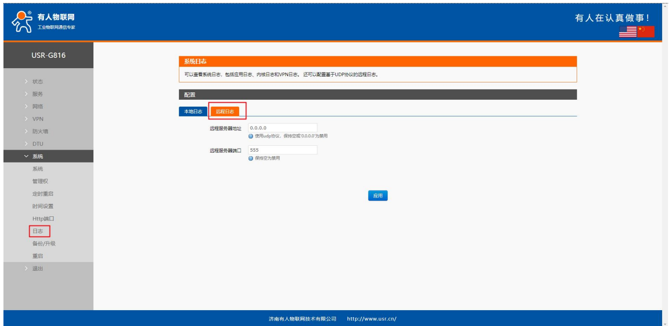
图 15 远程日志
