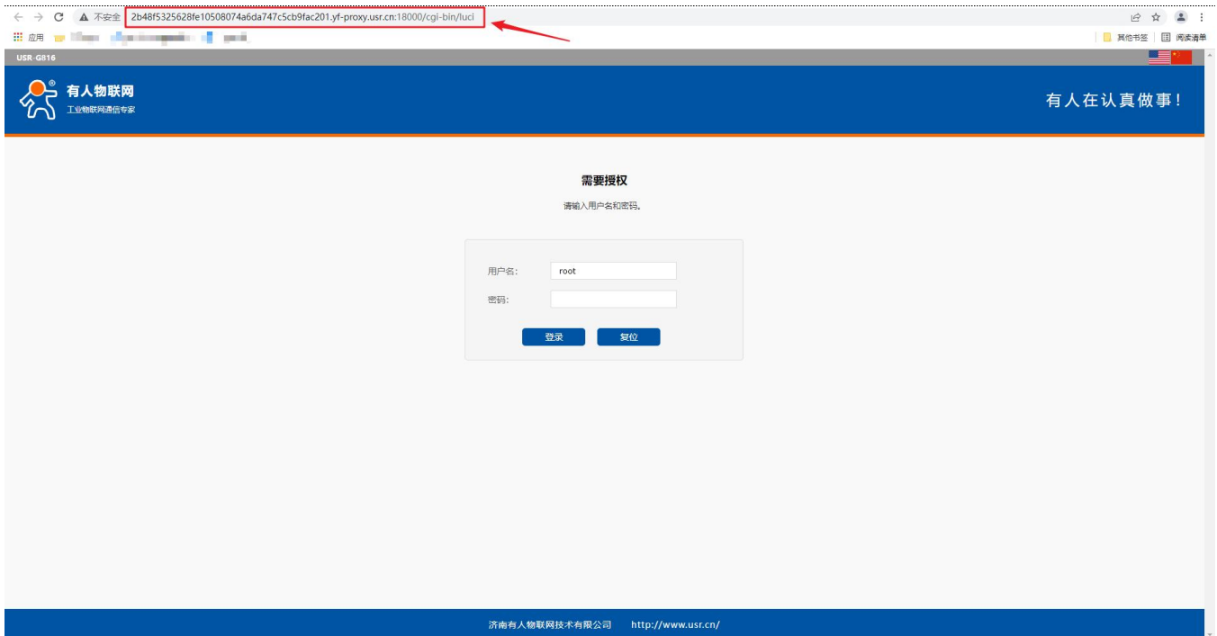
图 76 配置网页（二）
