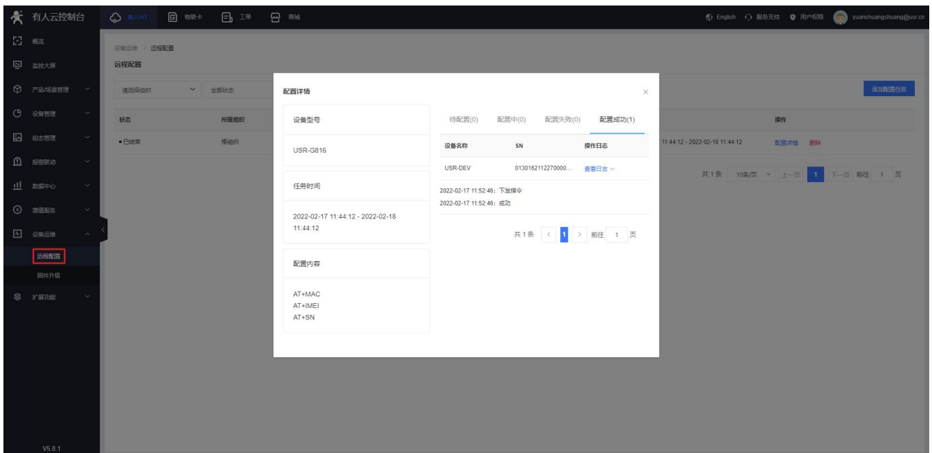
图 80 远程配置（四）
