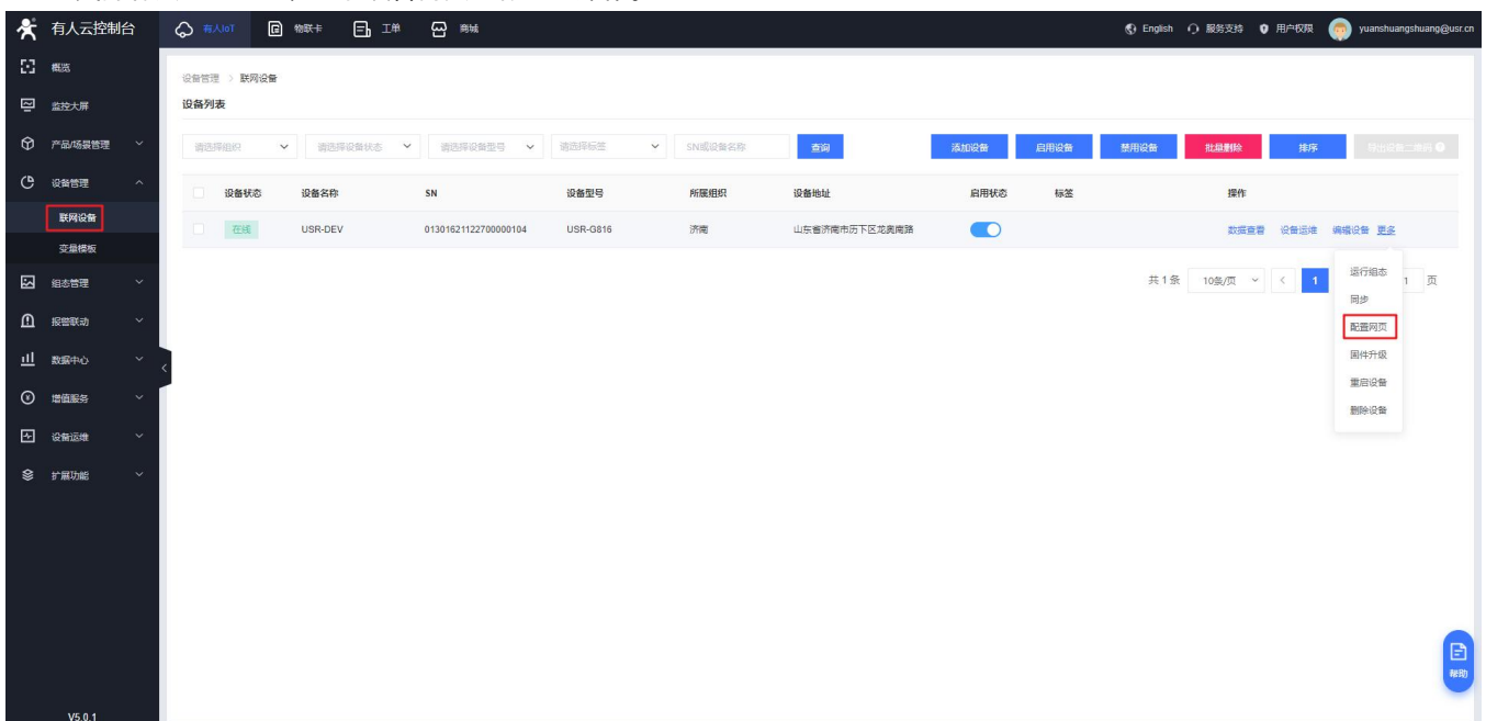
图 75 配置网页（一）
