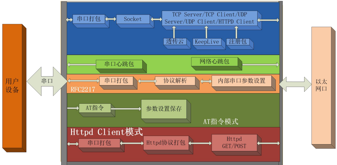
图 1. K6 功能框图
