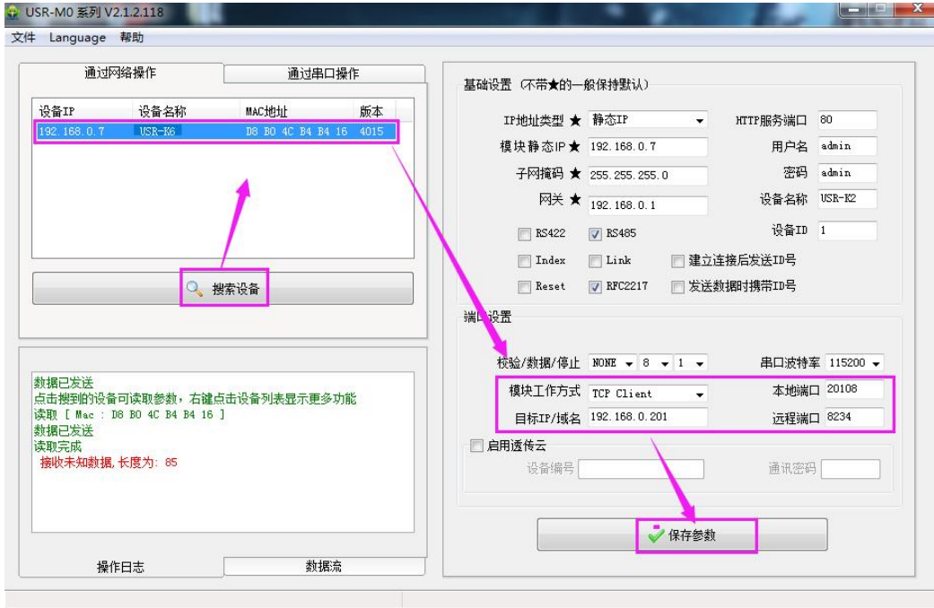
图 8. TCP Client 软件设置
