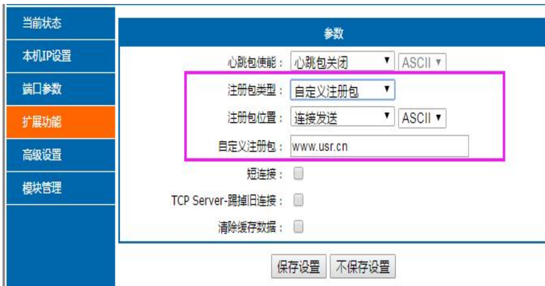
图 31. 注册包功能
