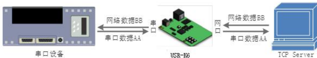
图 7. TCP Client 模式说明
