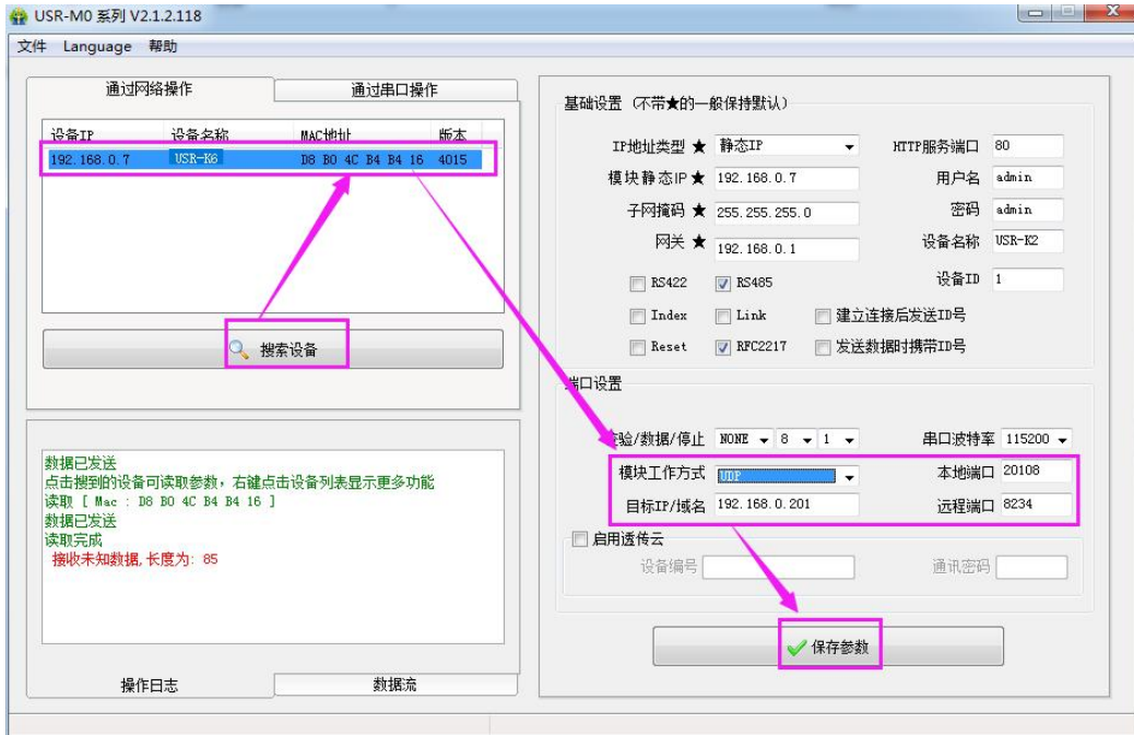
图 16. UDP Client 软件设置
