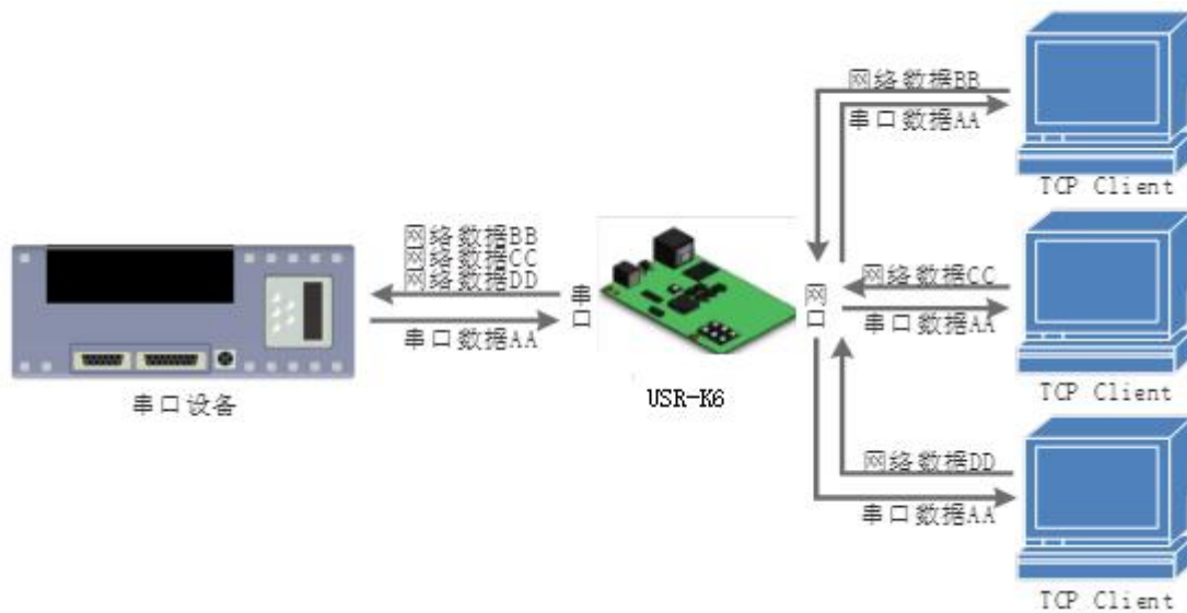
图 11. TCP Server 模式说明
