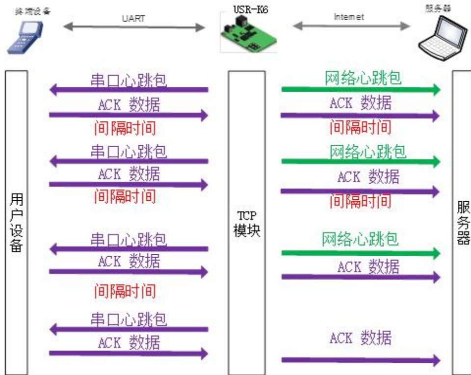
图 28. 心跳包功能示意图
