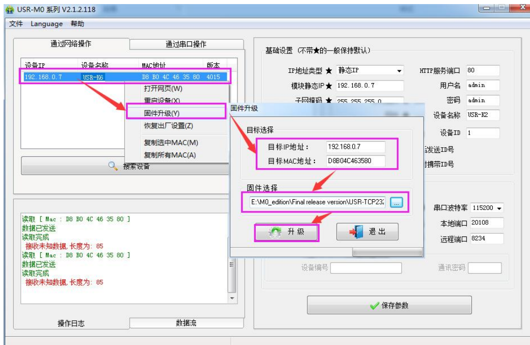
图 5. 选择固件
