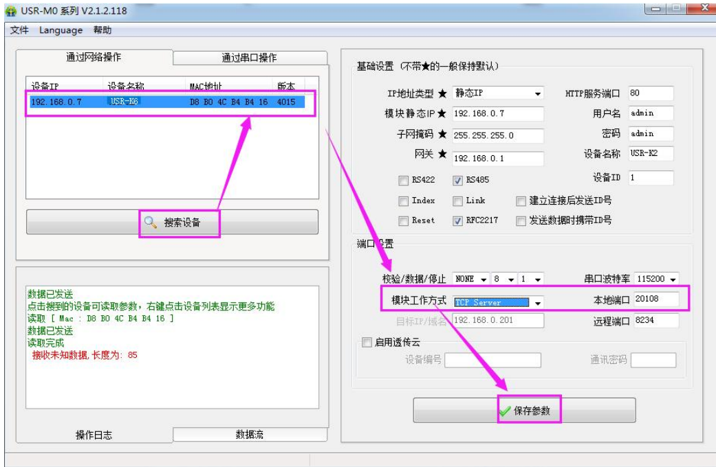
图 12. TCP Server 软件设置图
