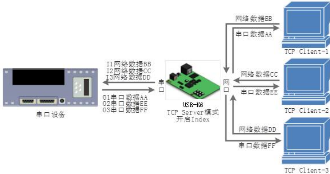
图 34. Index 功能示意图
