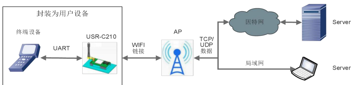
图 5 模块基本功能
