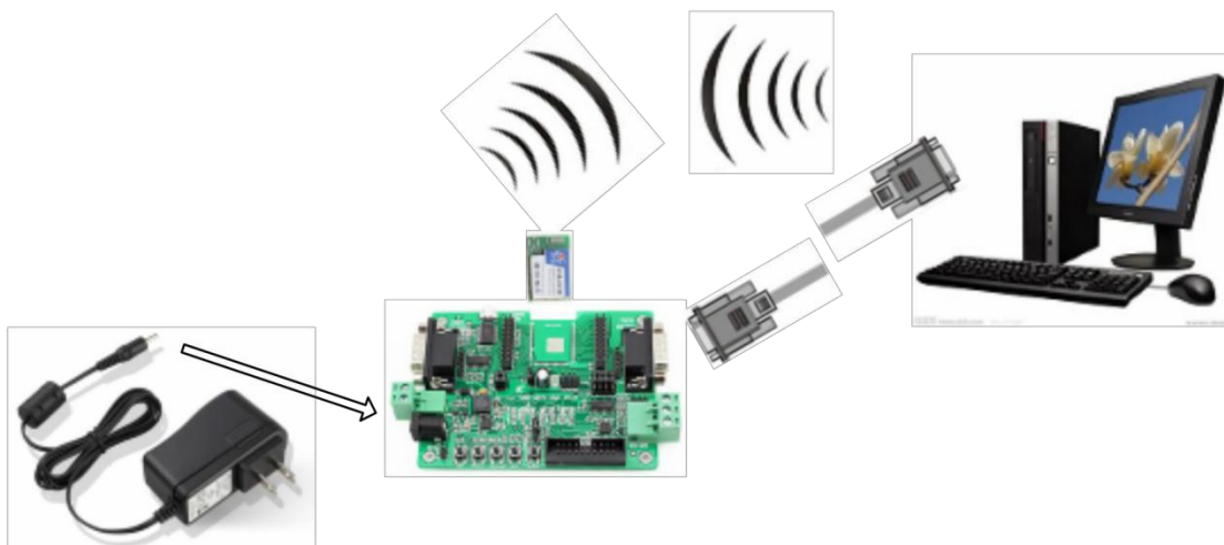
图 2 硬件连接图
