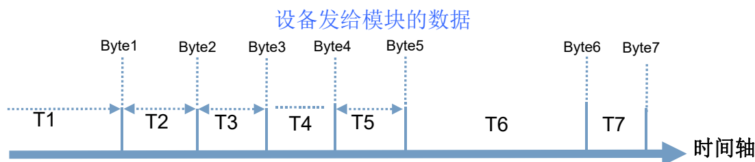
图 18 切换指令模式时序
