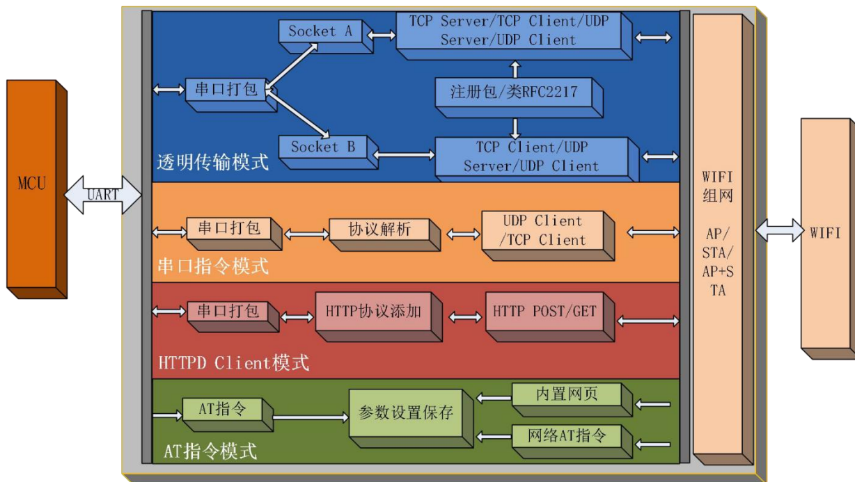
图 8 功能框图
