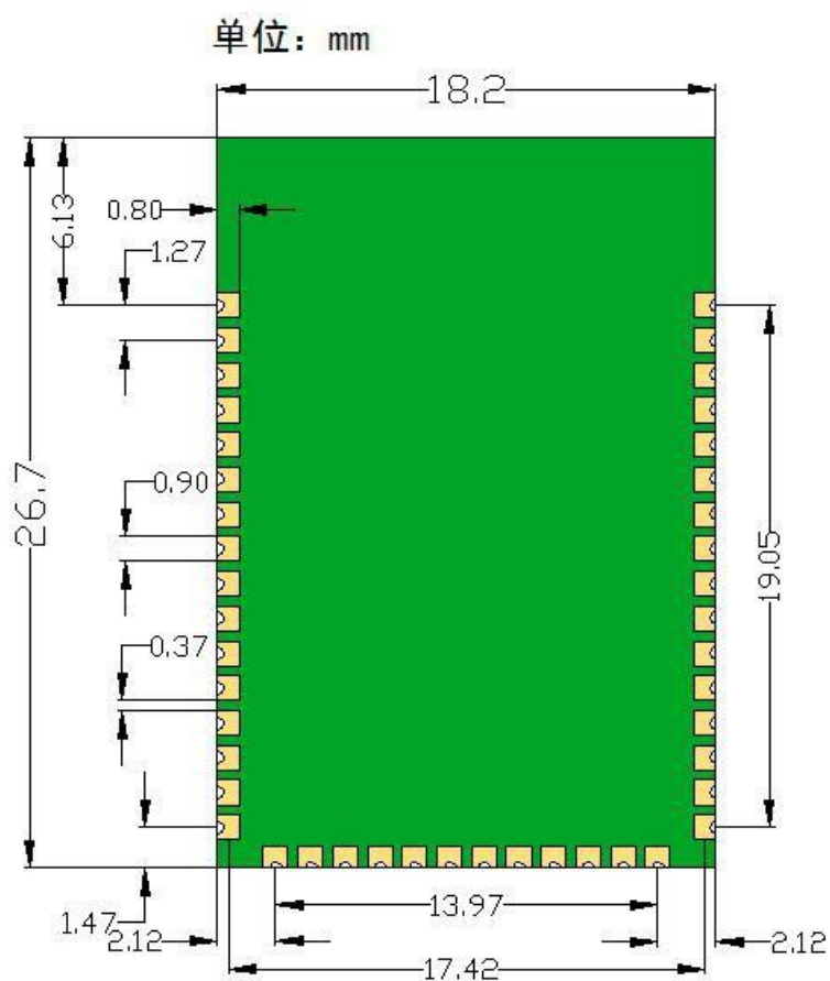
图 7 USR-C210 引脚图
