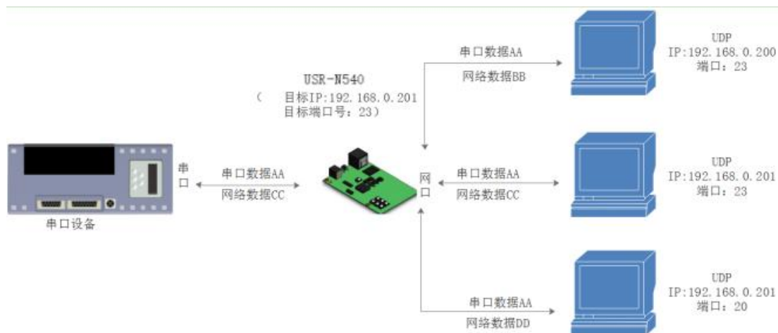
图 21 UDP Client 模式说明
