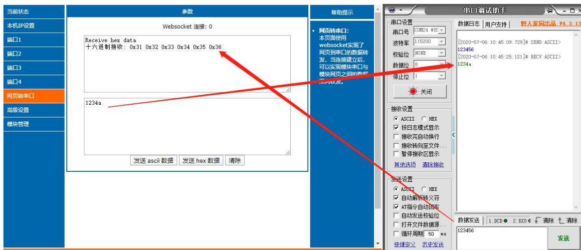
图 33 网页转串口收发数据展示
