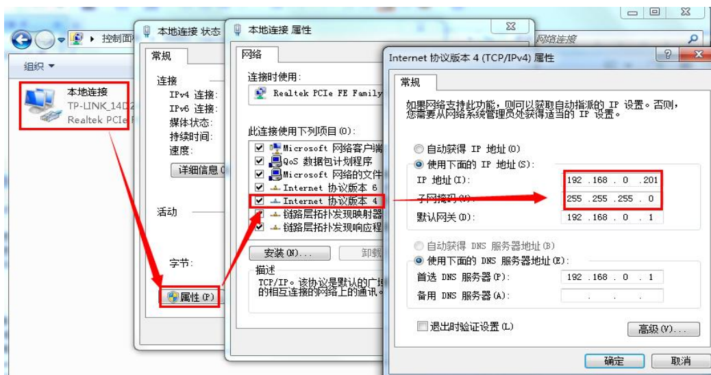
图 3 PC 机本地连接设置
