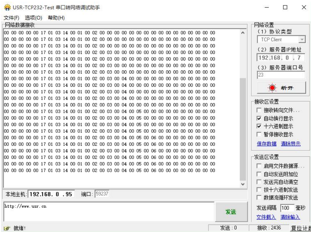
图 52 Modbus RTUS 主动查询设置截图
