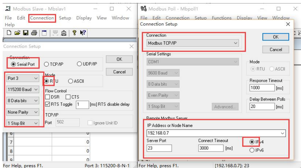
图 48 Modbus RTU 转 Modbus TCP 软件设置截图
