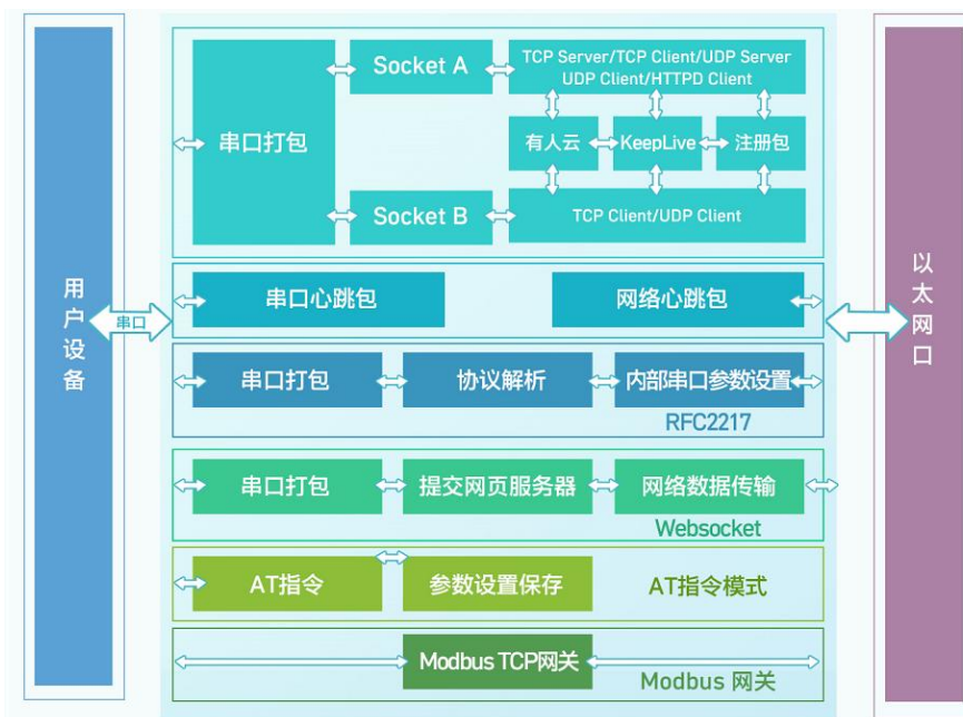
图 7 N540 功能框图
