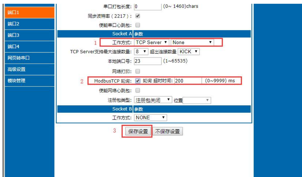
图 54 Modbus 轮询网页设置截图
