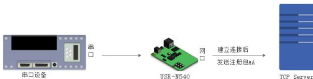
图 58 注册包建立连接发送注册包
