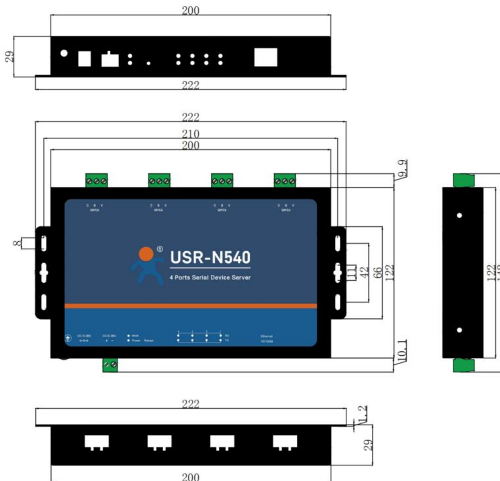
图 5 N540 尺寸图
