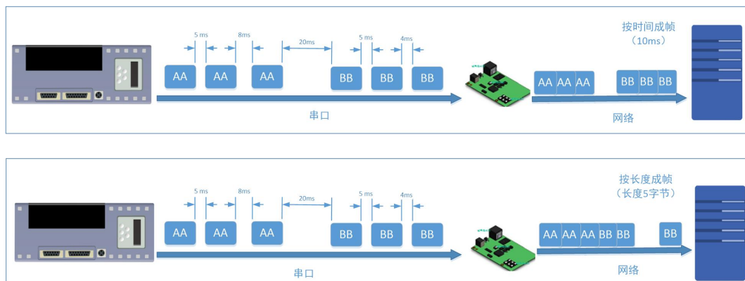
图 40 串口成帧说明
