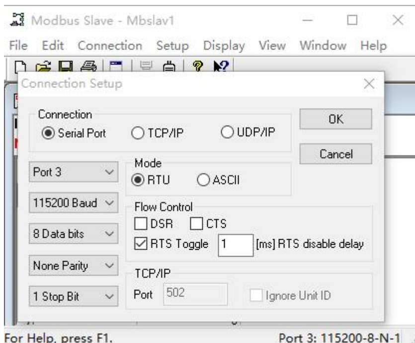
图 51 Modbus RTU 主动查询设置截图
