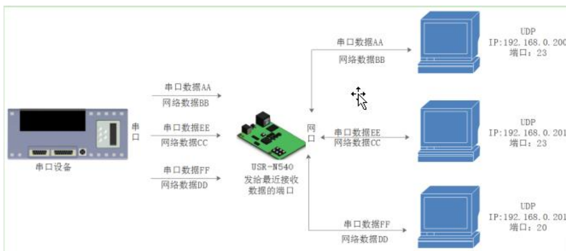
图 24 UDP Server 模式说明
