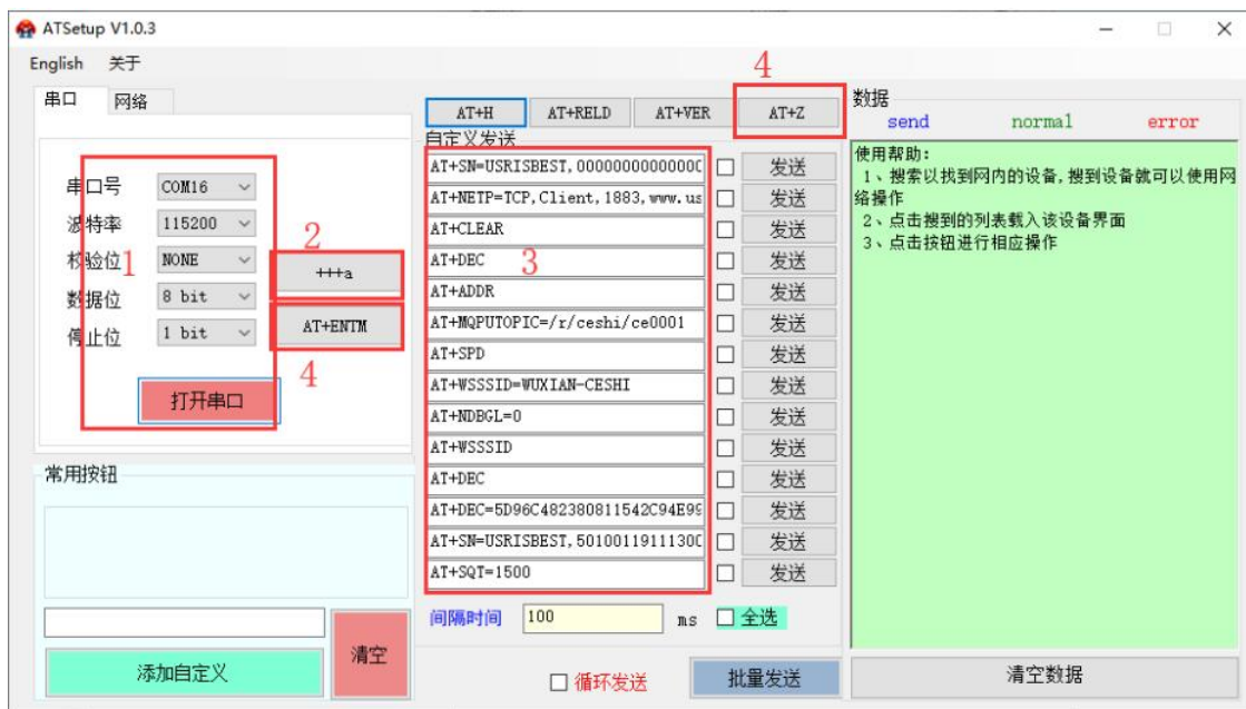
图 47 AT 指令设置软件
