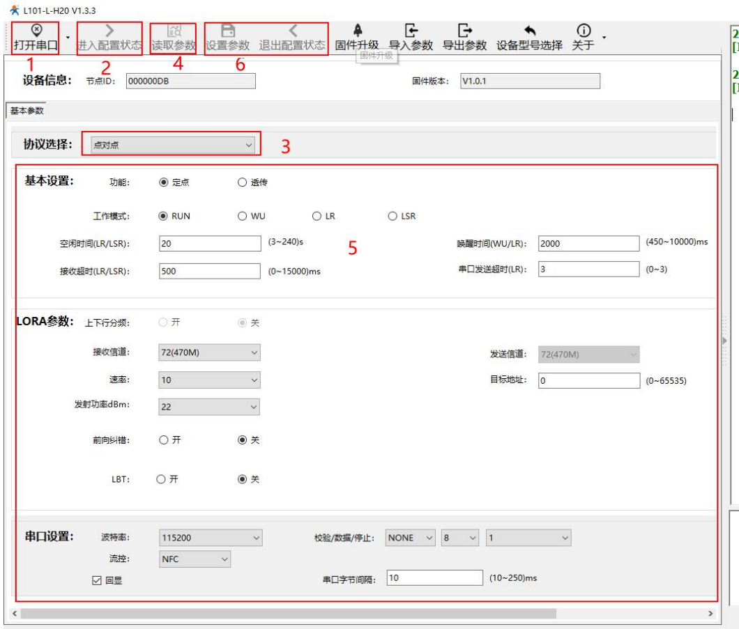
图 46 L101-L-H20 设置软件
