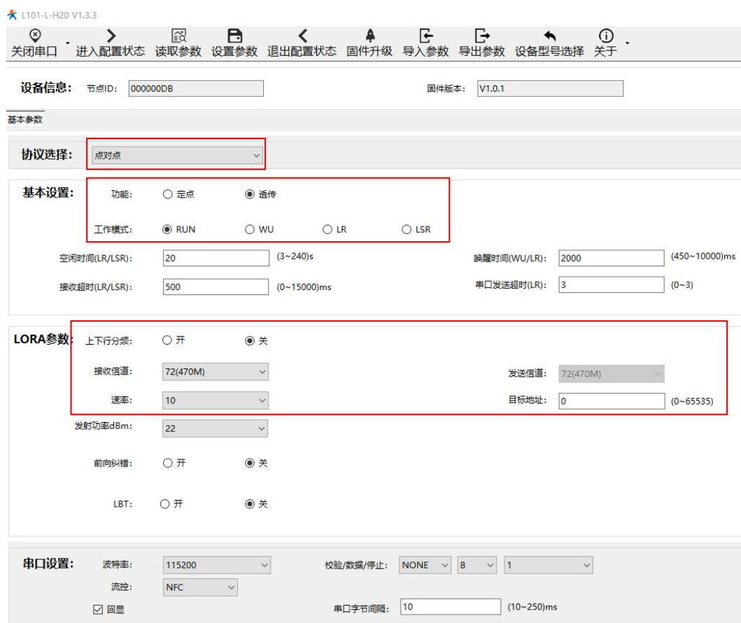
图 6 透明传输设置方法
