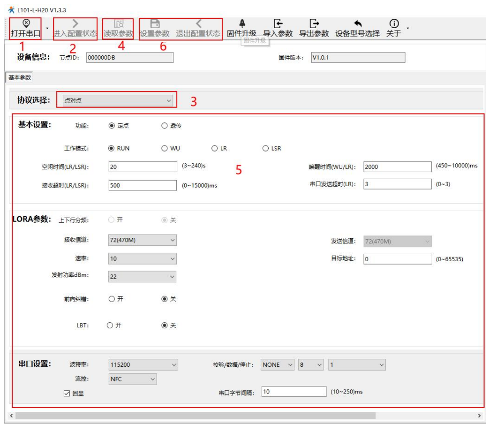
图 21 L101-L-H20 设置软件
