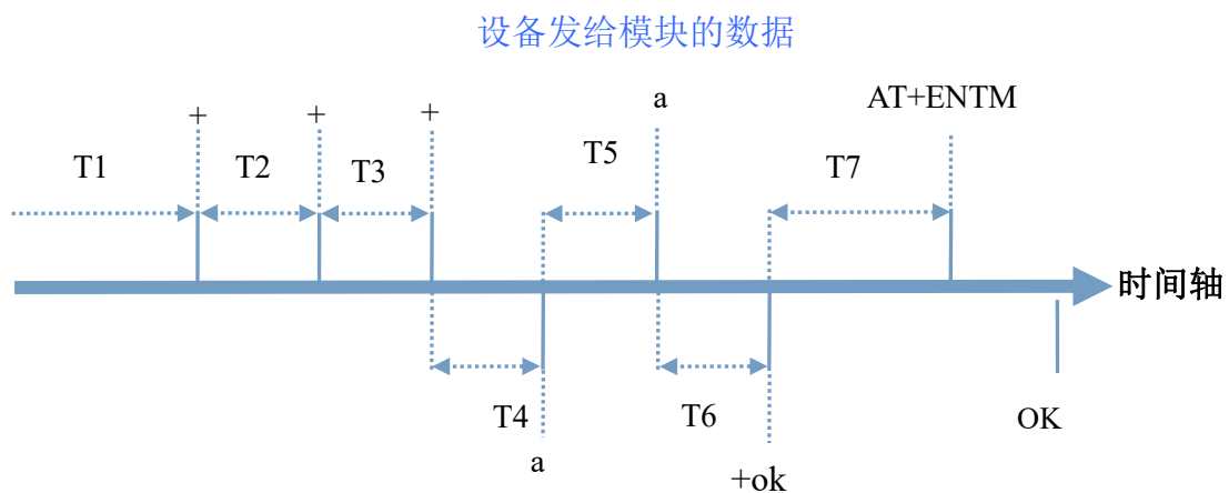
图 16. +++a 时序图
