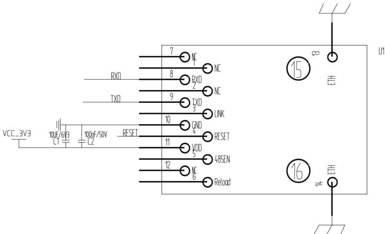
图 6 USR-K5 电源接口示意图
