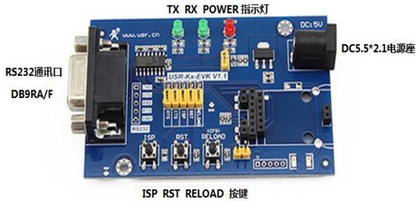
图 4 USR-Kx-EVK 示意图
