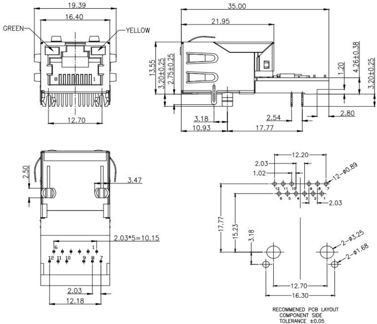
图 2 机械尺寸
