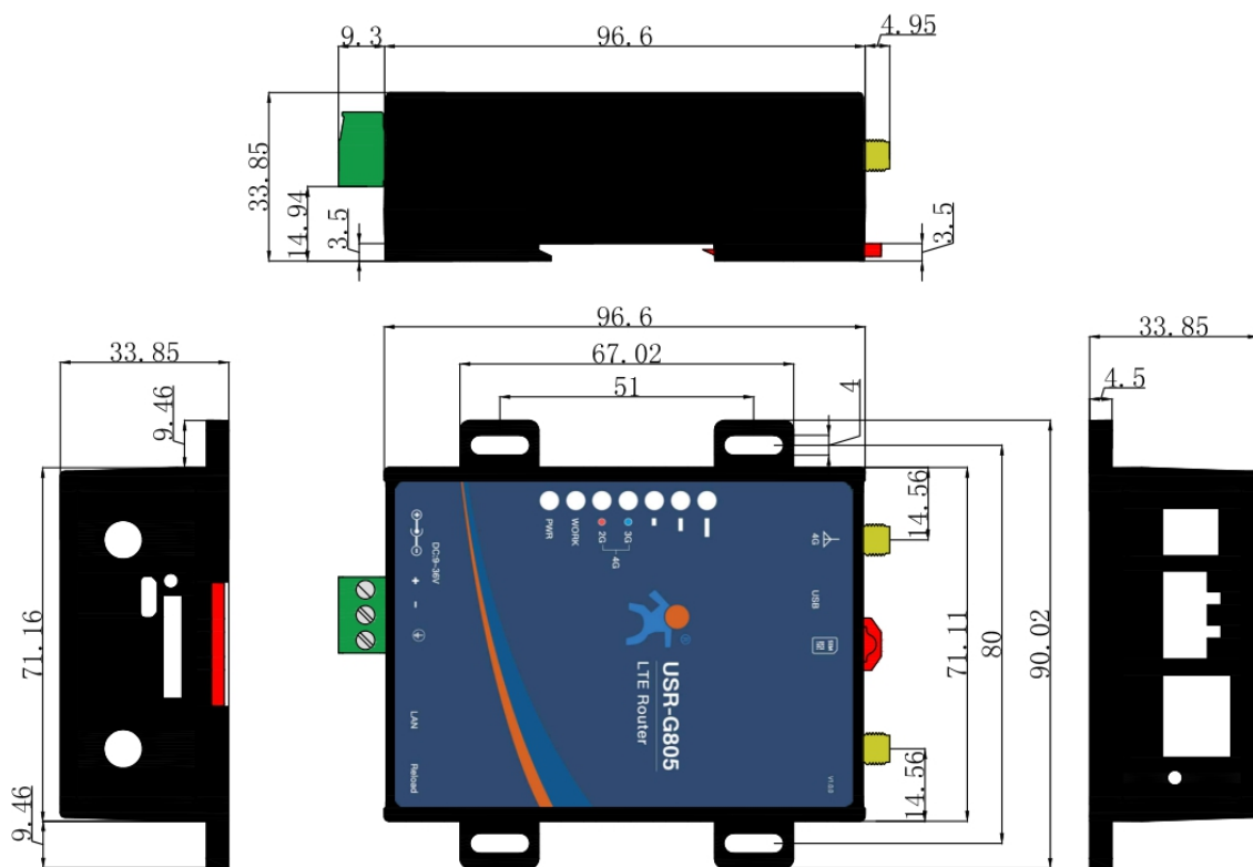
USR-G805 外观尺寸图 (单位: mm)
