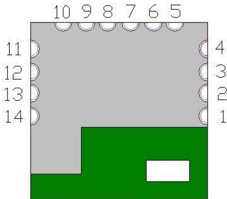
图 1 USR-BLE101 引脚图
