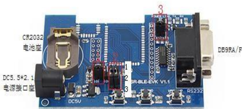
图 4 USR-BLE-EVK 模块评估板
