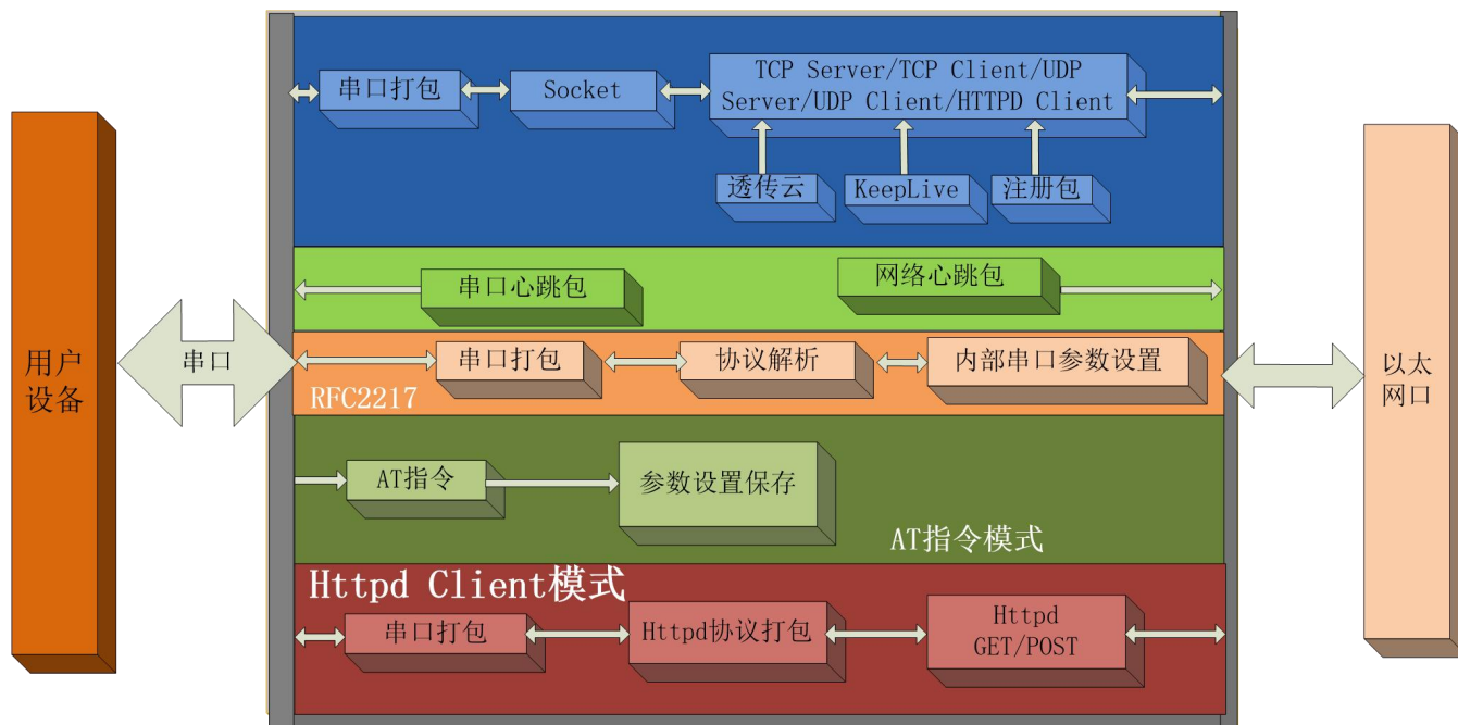
图 1. T2 功能框图
