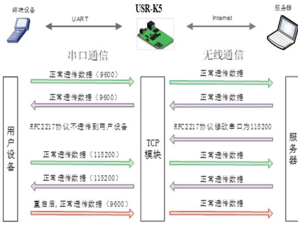
图 4.14 类 RFC2217 功能框图
