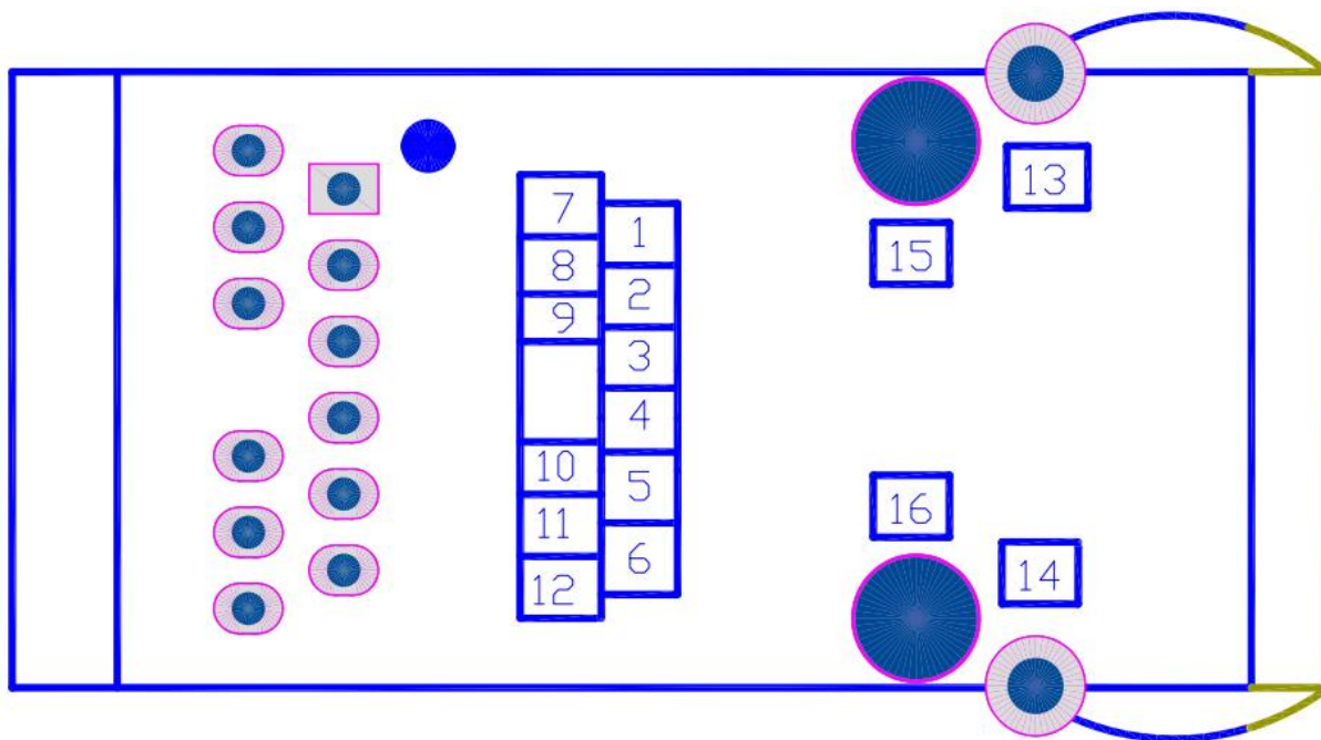
图 3 USR-K5 引脚正视图
