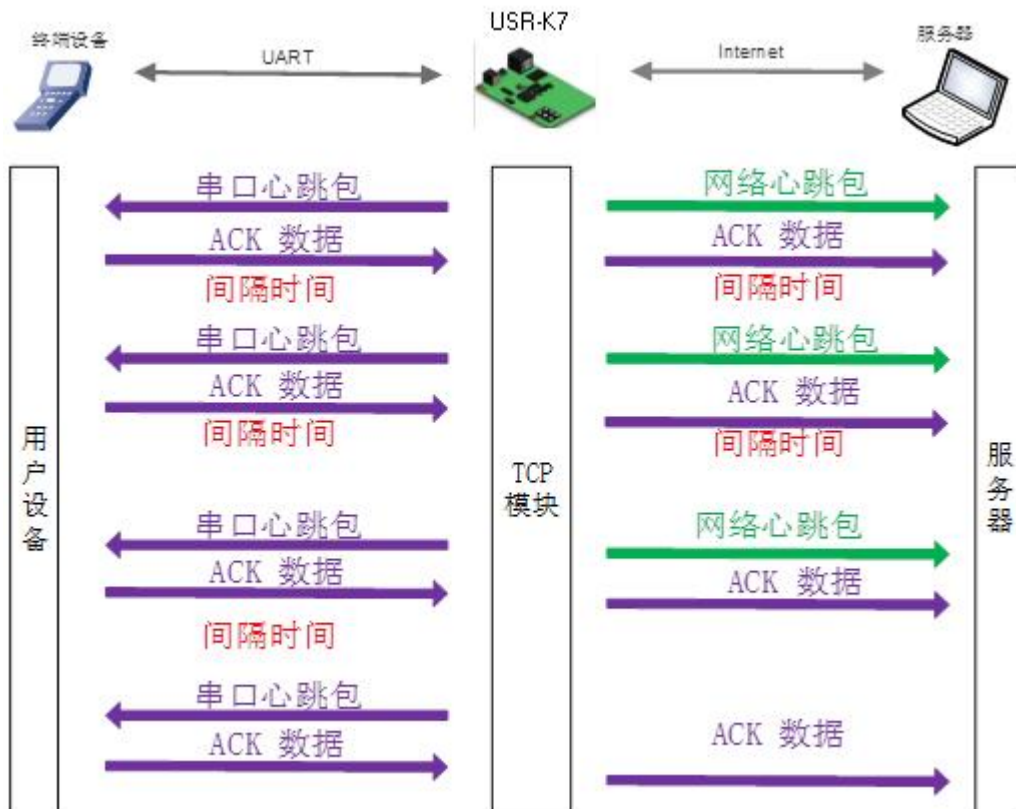
图 34 心跳包功能示意图
