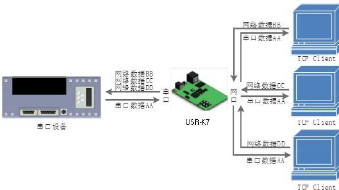
图 12 TCP Server 模式说明
