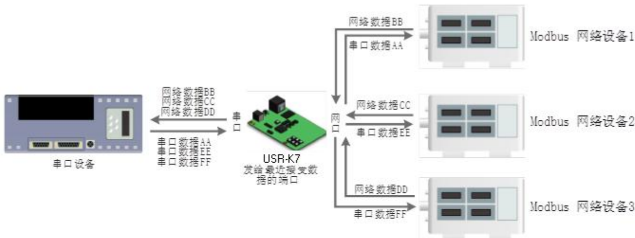
图 43 Modbus TCP
