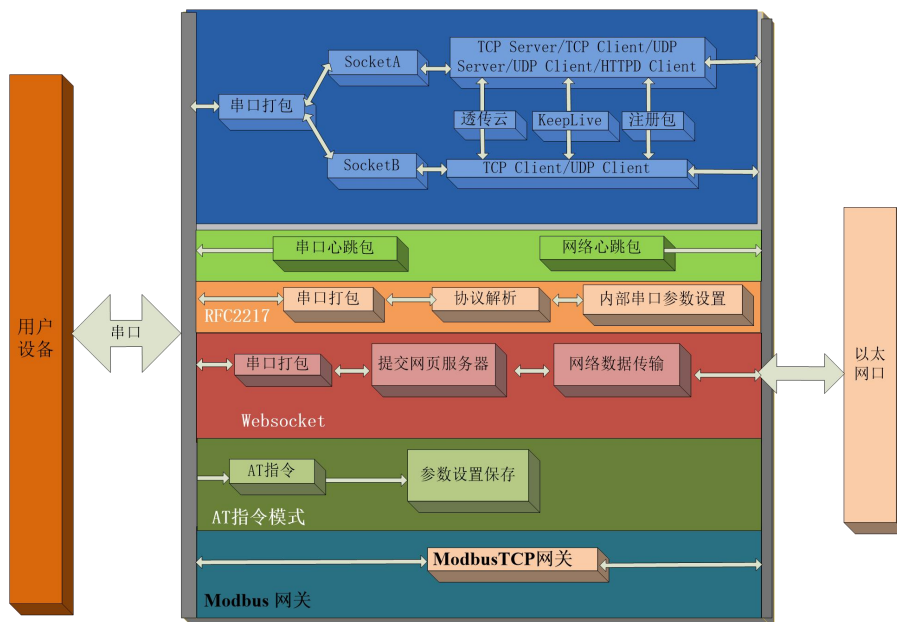
图 1 K7 功能框图
