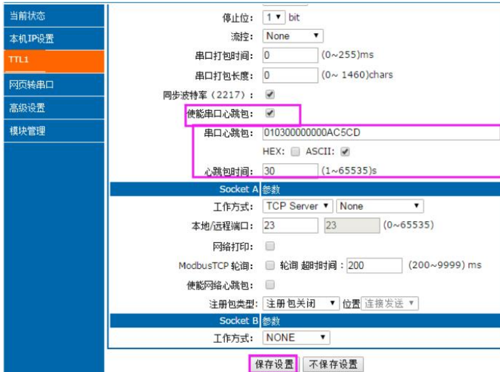
图 40 Modbusrtu 主动查询设置截图
