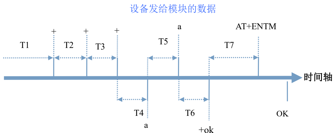
图 16. +++a 时序图
