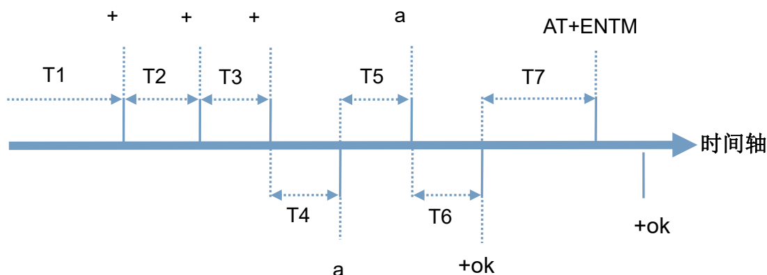
图 55 进入串口 AT 命令模式时序
