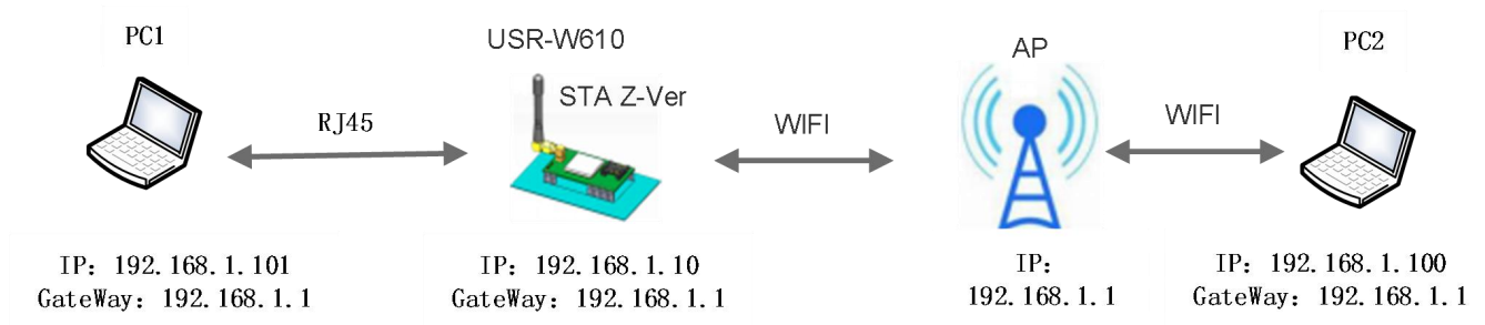
图 12 有线加无线组网应用（桥接）
