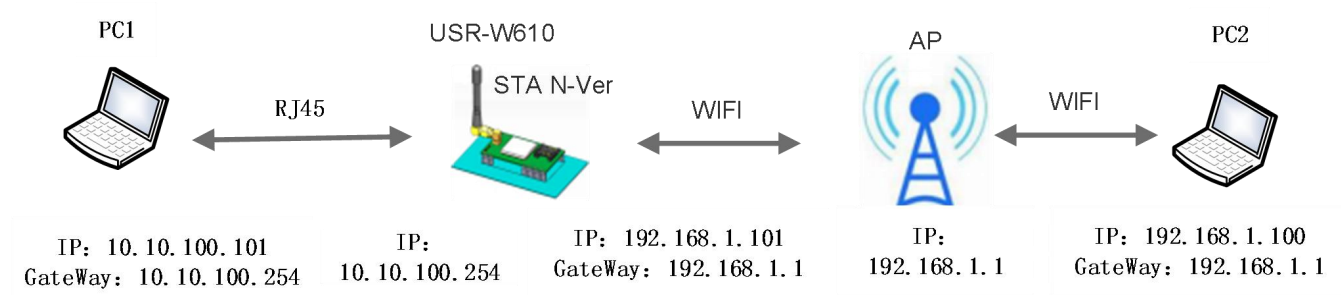
图 10 有线加无线组网应用（路由）
