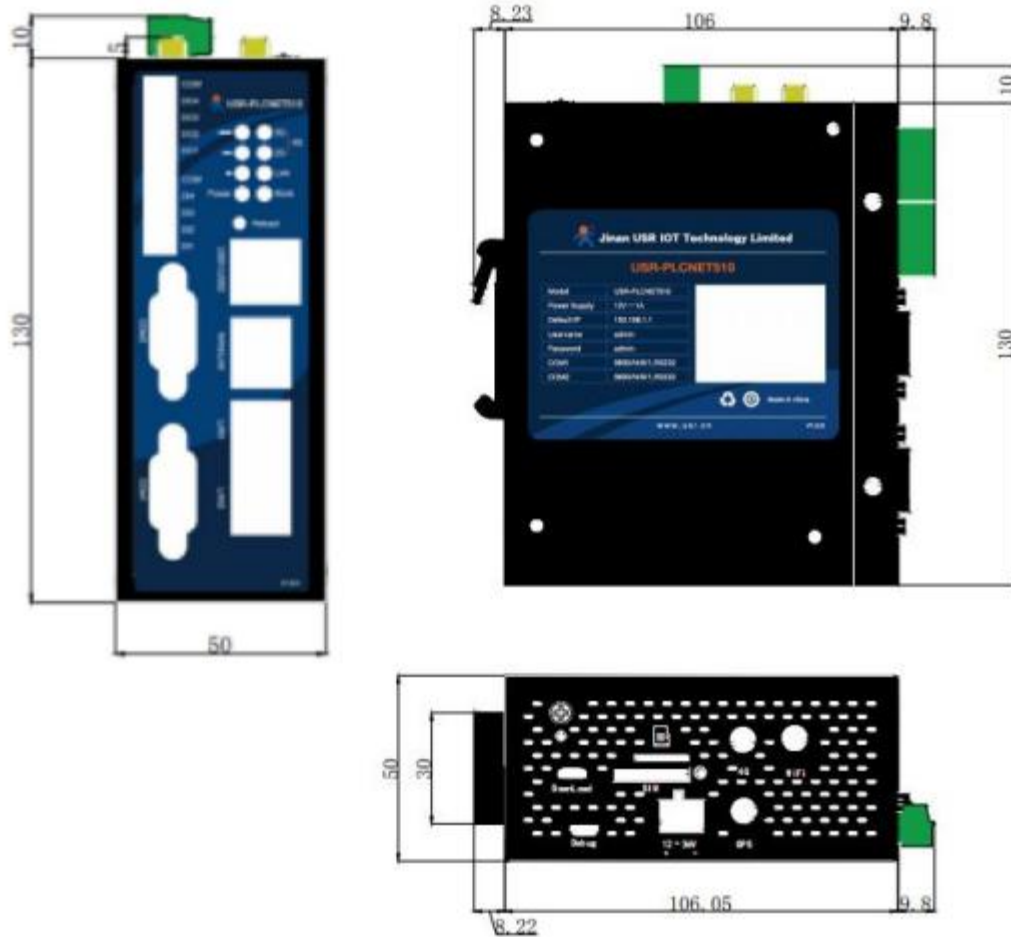
PLCNET510外观尺寸图
