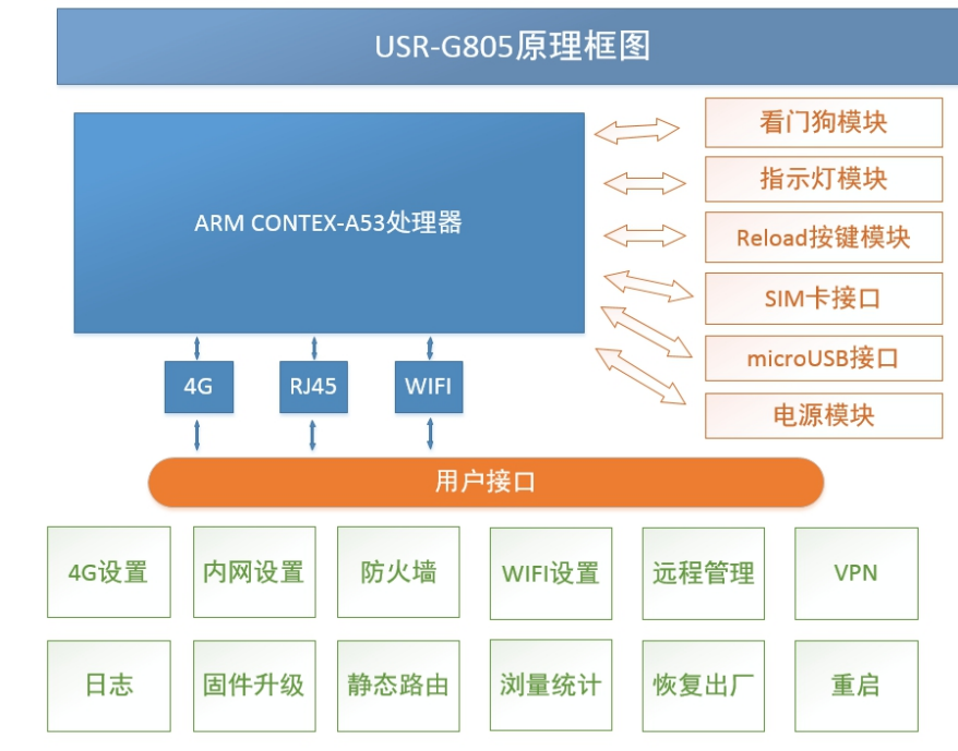
图 2 功能框图
