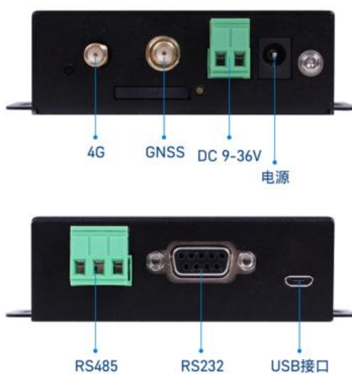
图 2. USR-G780s 接口图
