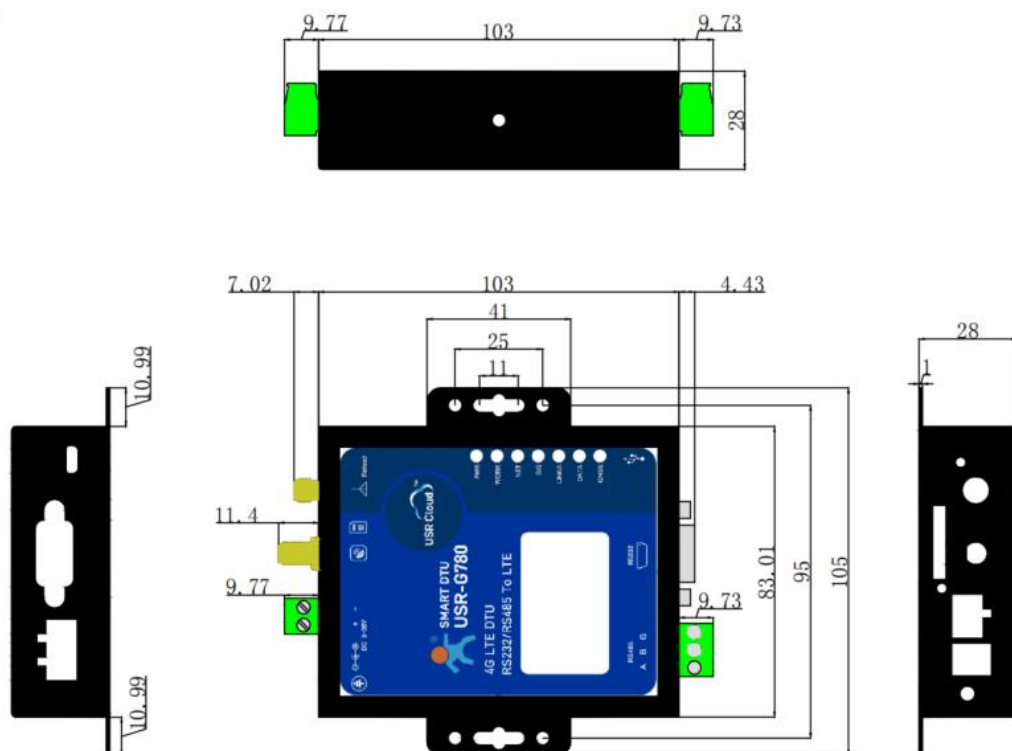
图 1. USR-G780s 尺寸图
