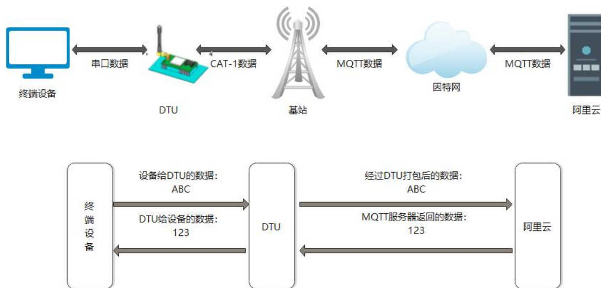
图 1. MQTT 模式
