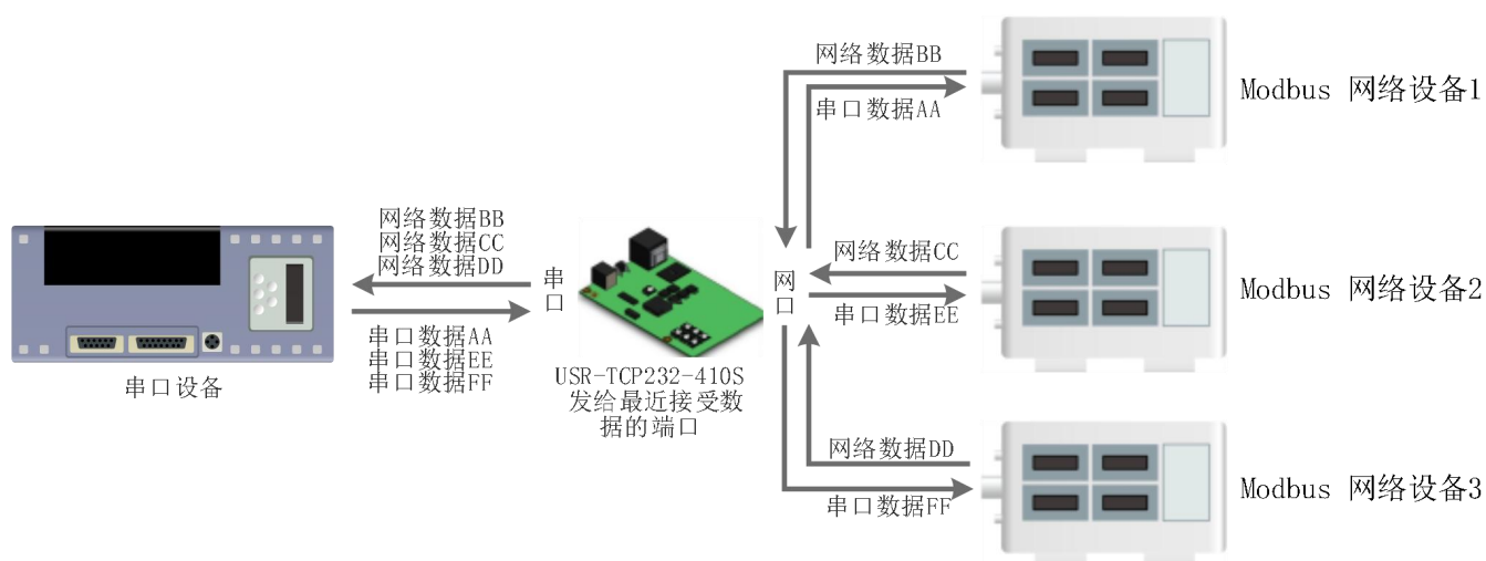
图 45 Modbus 多主机轮询
