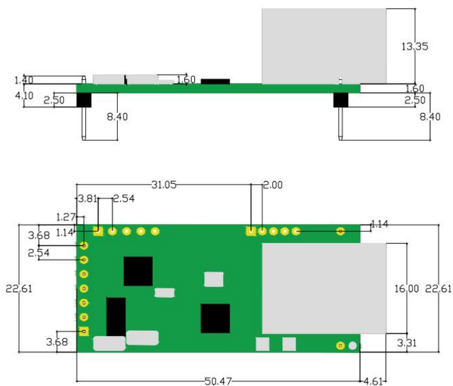
图 7 尺寸图
