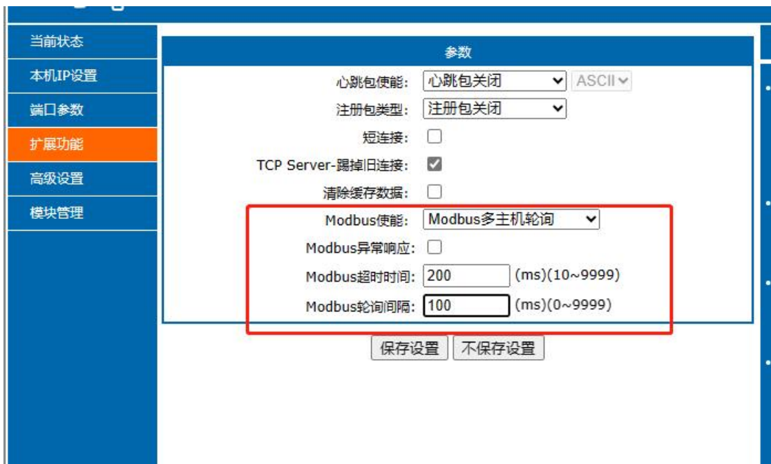
图 46 Modbus 轮询网页设置截图
