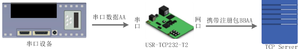
图 26 数据携带注册包
