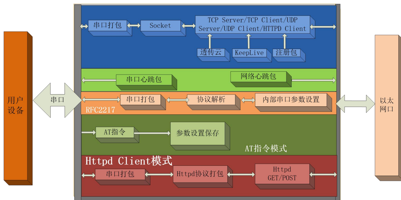
图 8 T2 功能框图
