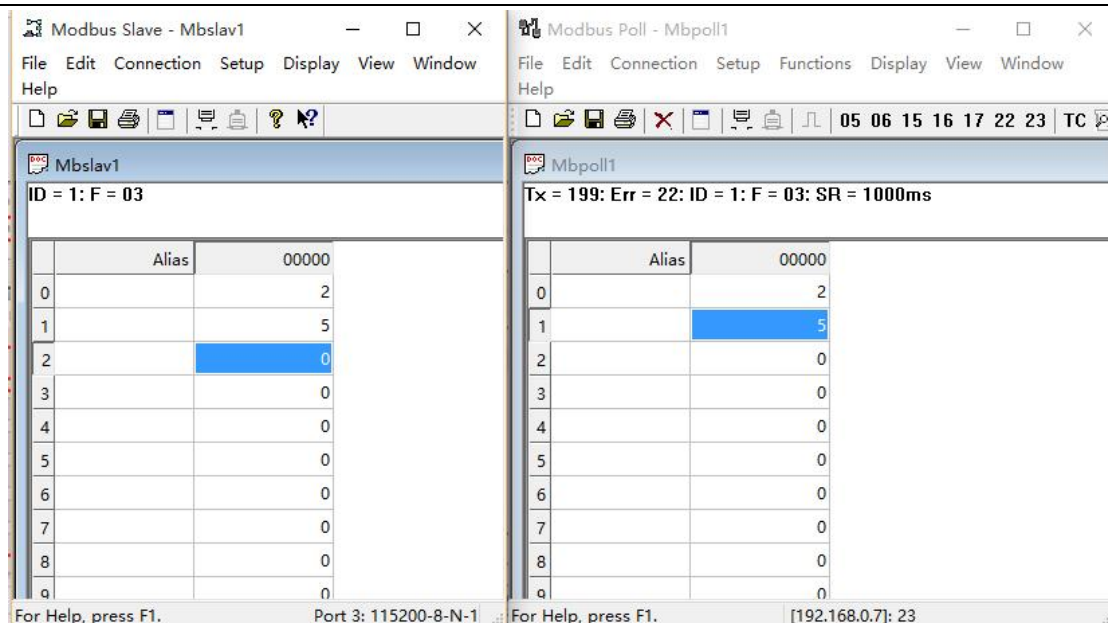
图 44 Modbus RTU 转 Modbus TCP 转换结果
