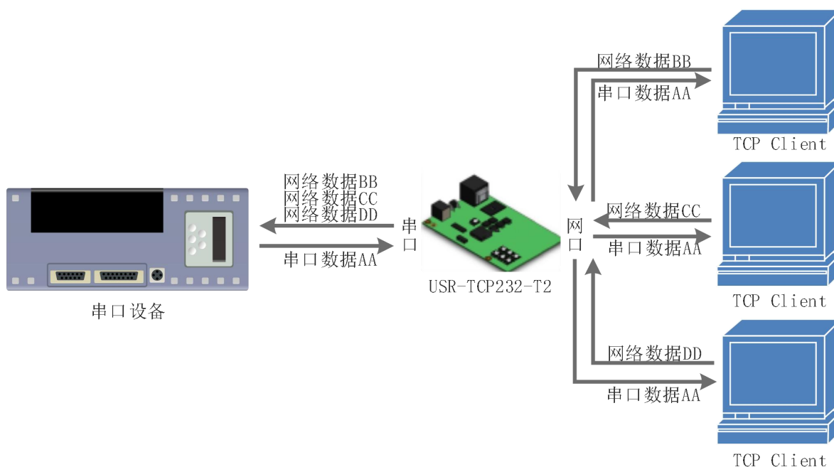
图 14 TCP Server 模式说明
