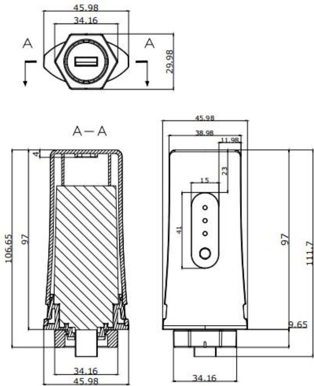
图 3. 尺寸图
