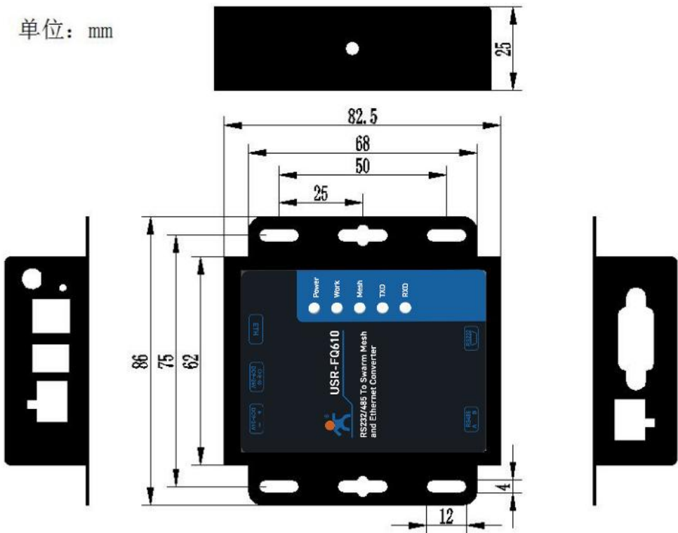
图 1 USR-FQ610 尺寸图
