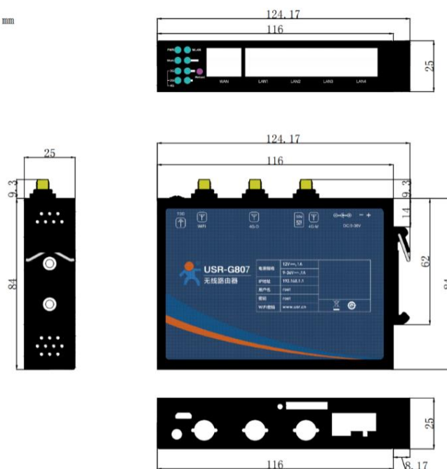
USR-G807 产品尺寸
