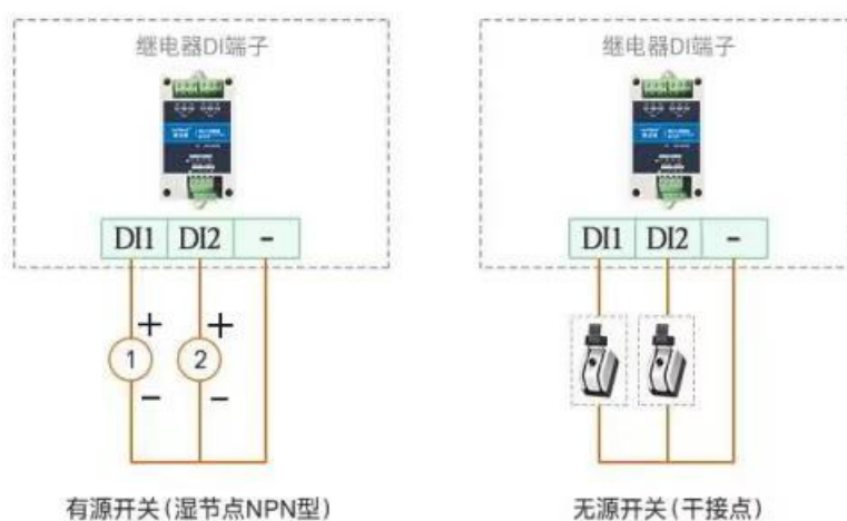
LH-IO222, 接有源NPN型开关、无源开关
