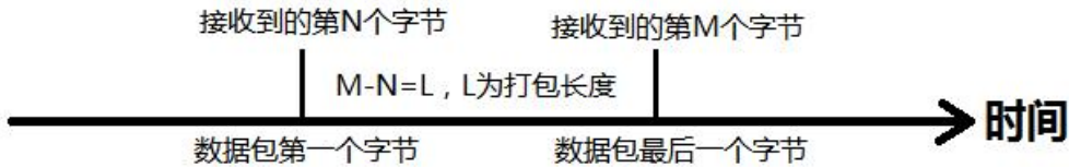
图 49. 长度触发模式
