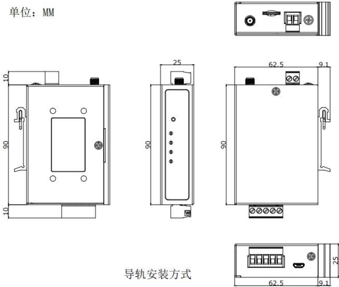
图 1. 导轨安装尺寸图
