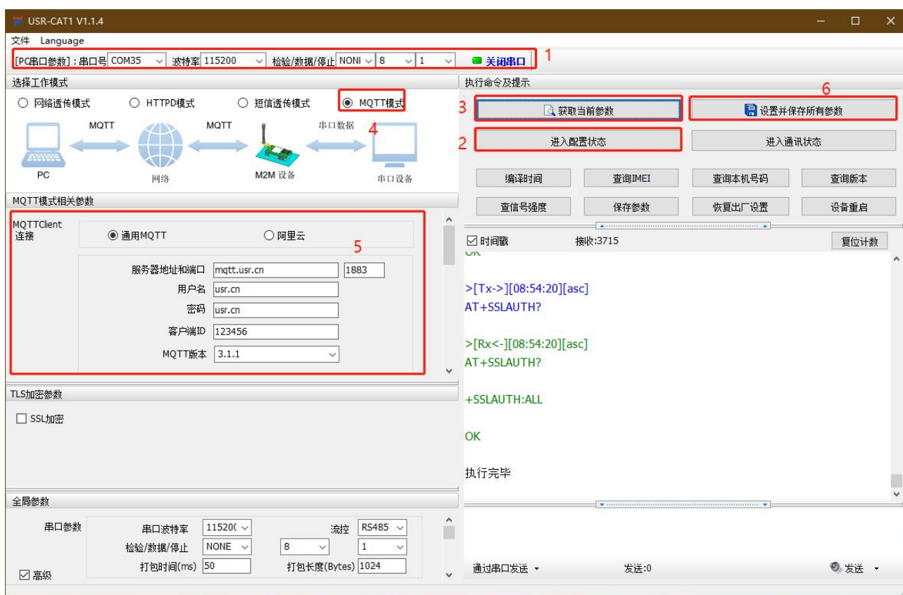
图 6. MQTT 基本参数配置
