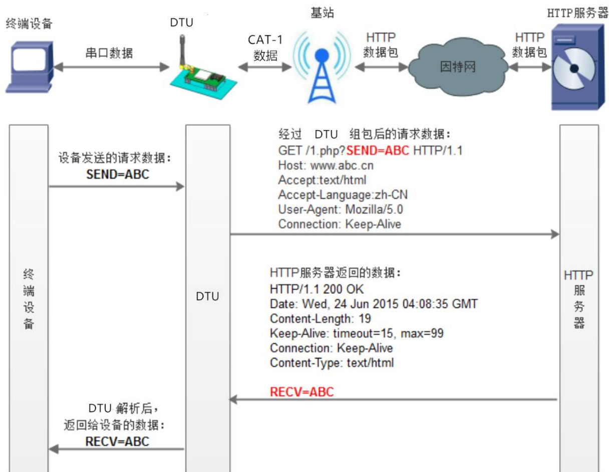
图 38. HTTPD Client 模式
