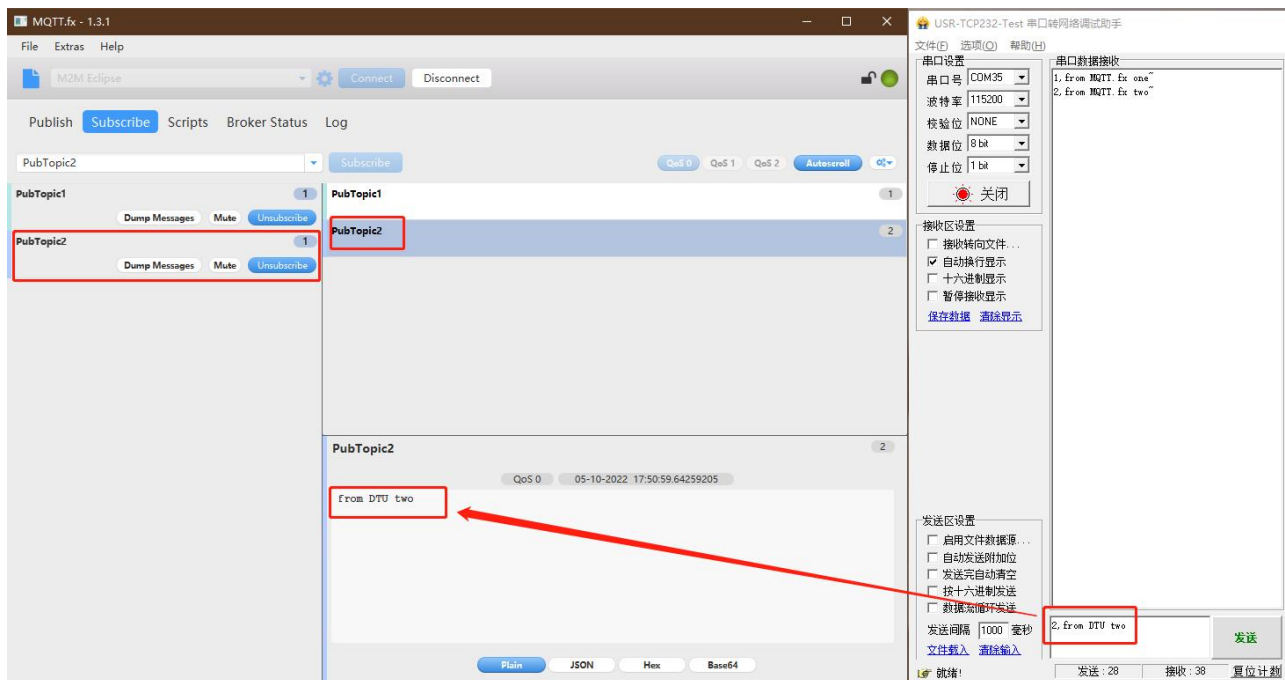
图 16. MQTT 推送数据测试 2
