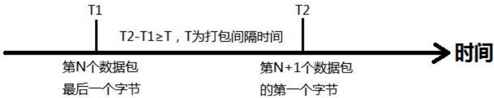
图 48. 时间触发模式
