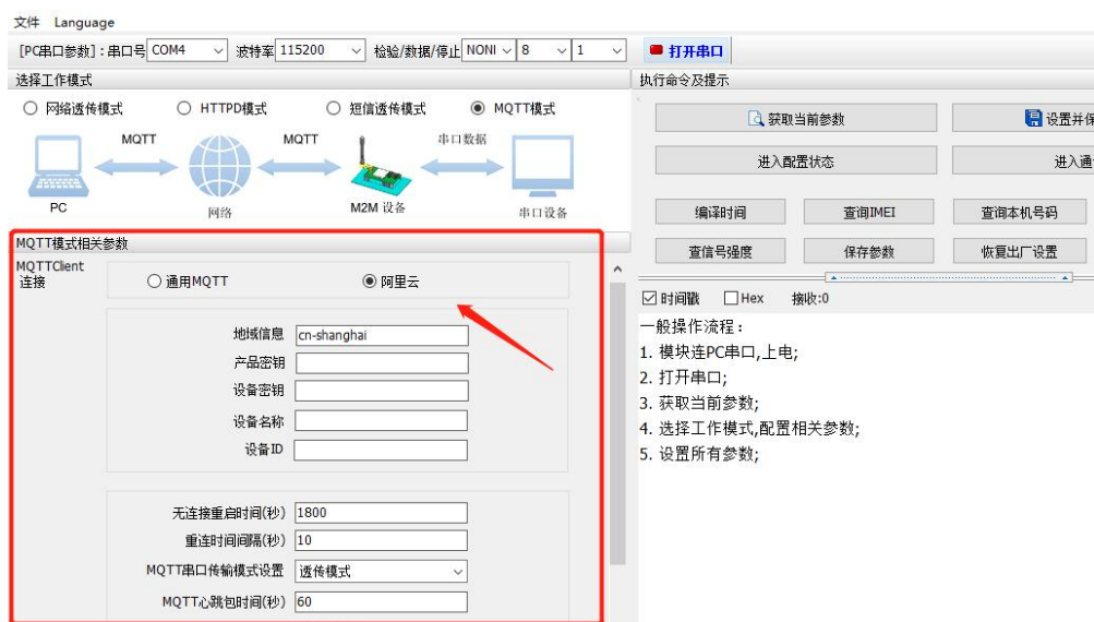
图 17. MQTT 模式阿里云接入示意图
