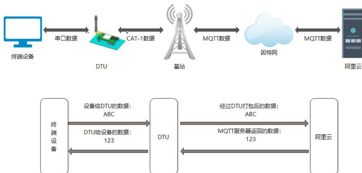
图 4. MQTT 模式
