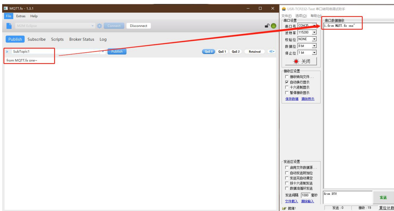
图 13. MQTT 订阅数据测试 1
