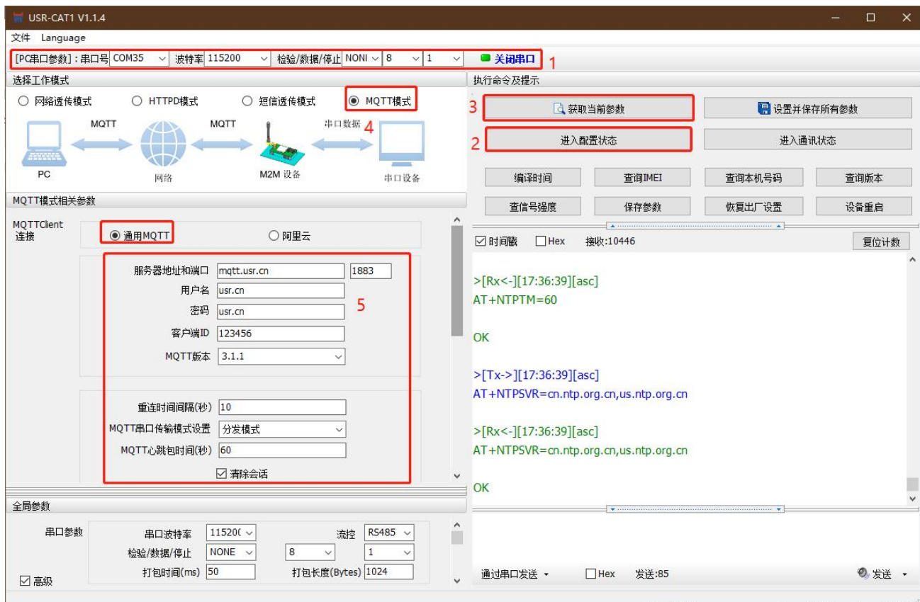
图 10. MQTT 基本参数设置
