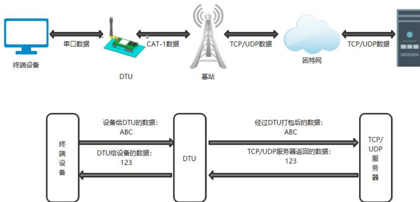
图 34. 网络透传模式
