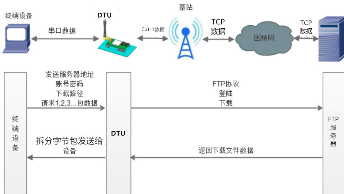
图 42. FTP 他升级协议示意图
