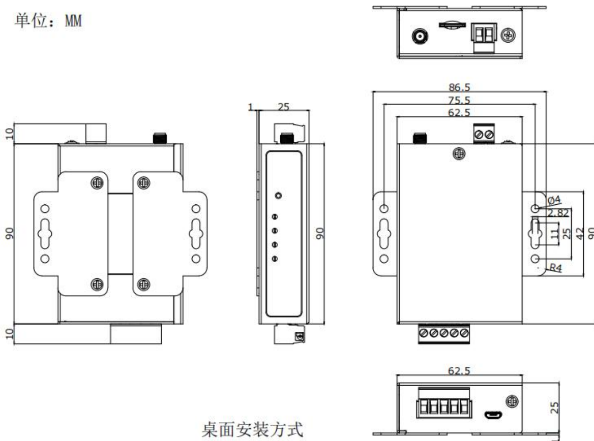
图 2. 挂耳安装尺寸图
