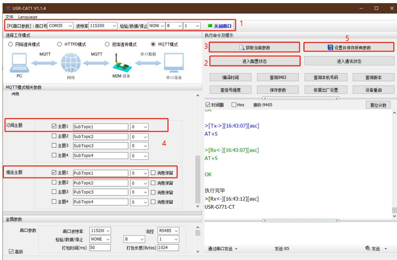
图 7. MQTT 主题配置
