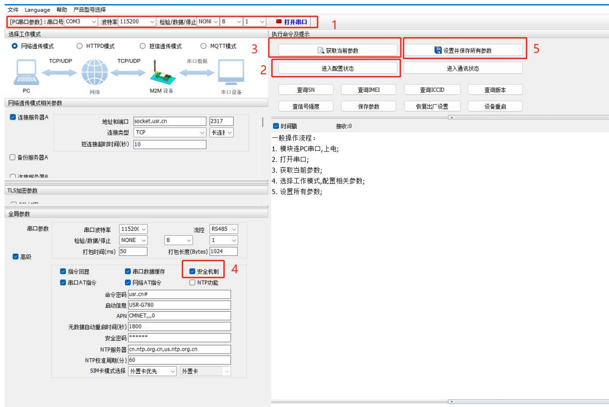
图 40. 设置软件示意图
