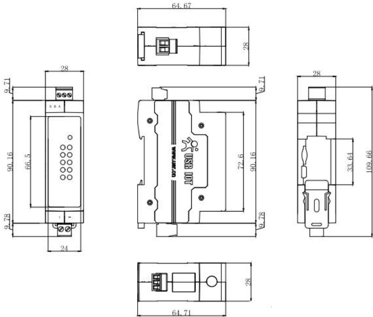
图 4 尺寸图
