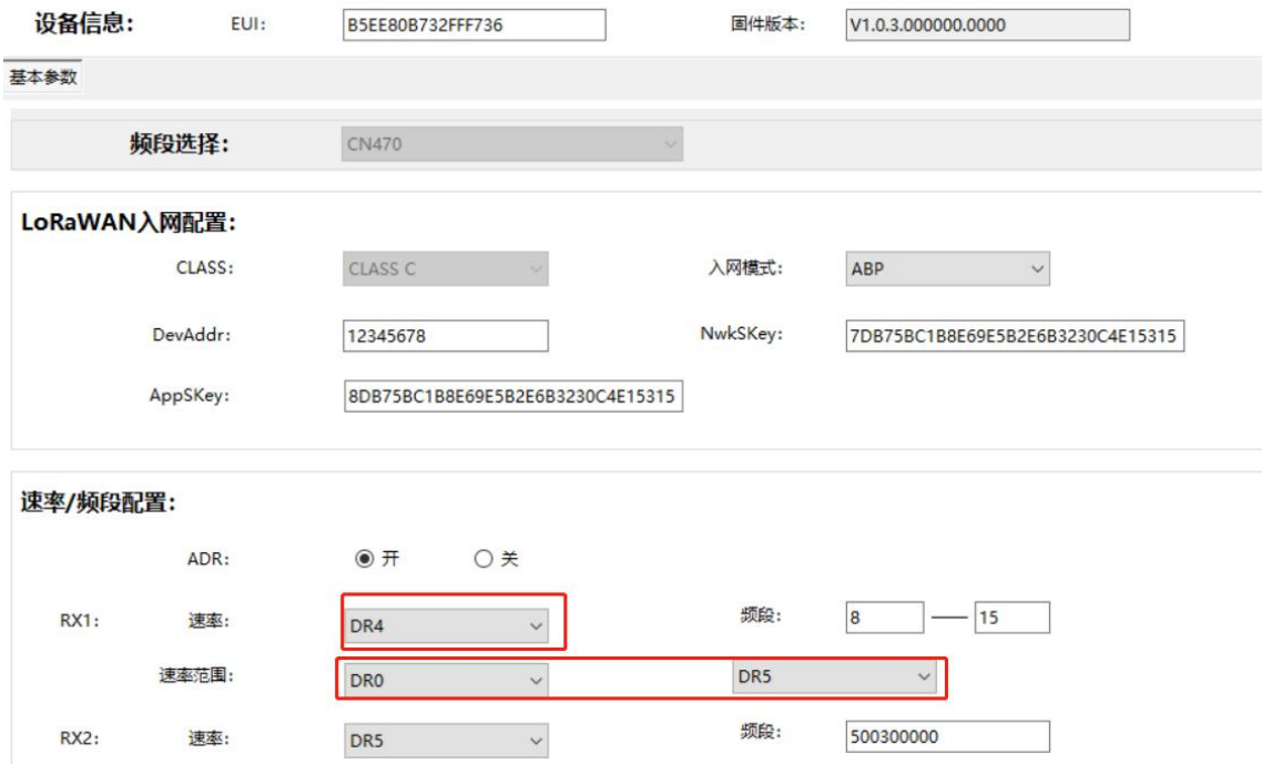
图 8 节点设置 RX1
