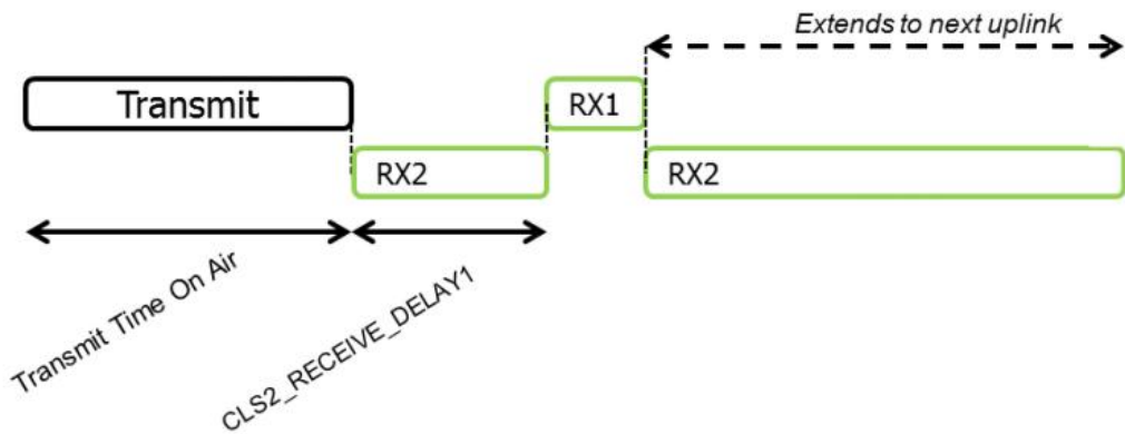
图 6 Class C 设备的通信机制
