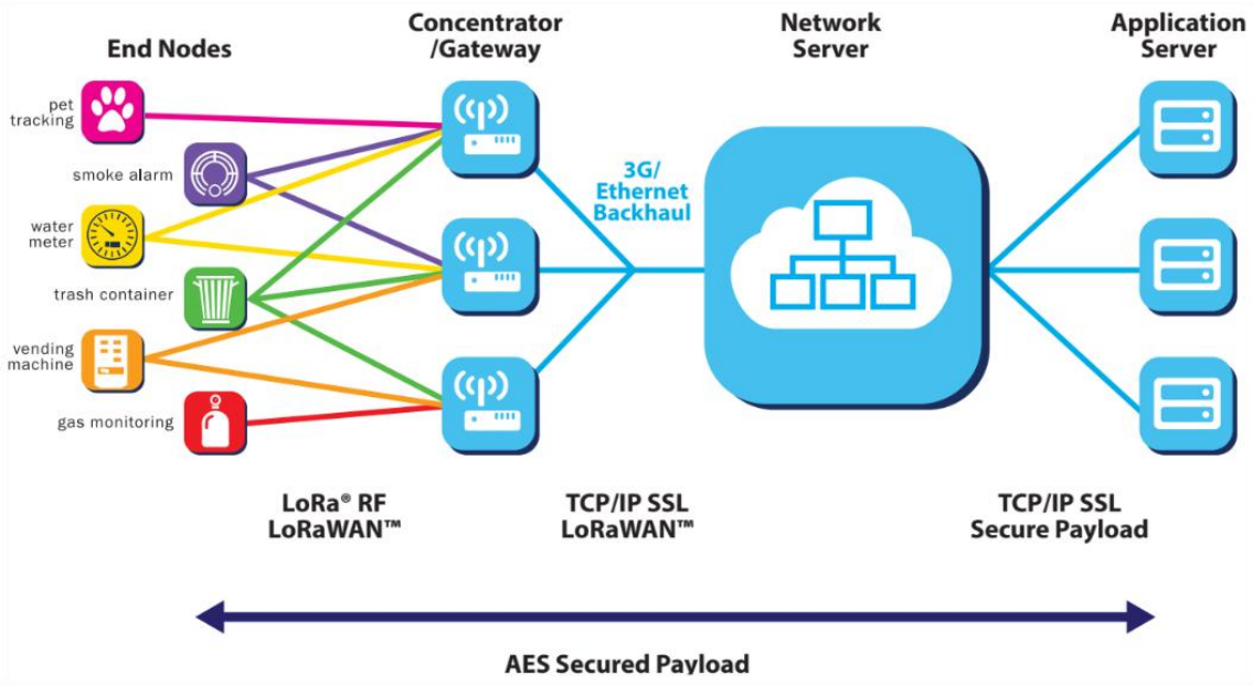
图 2 网络结构
