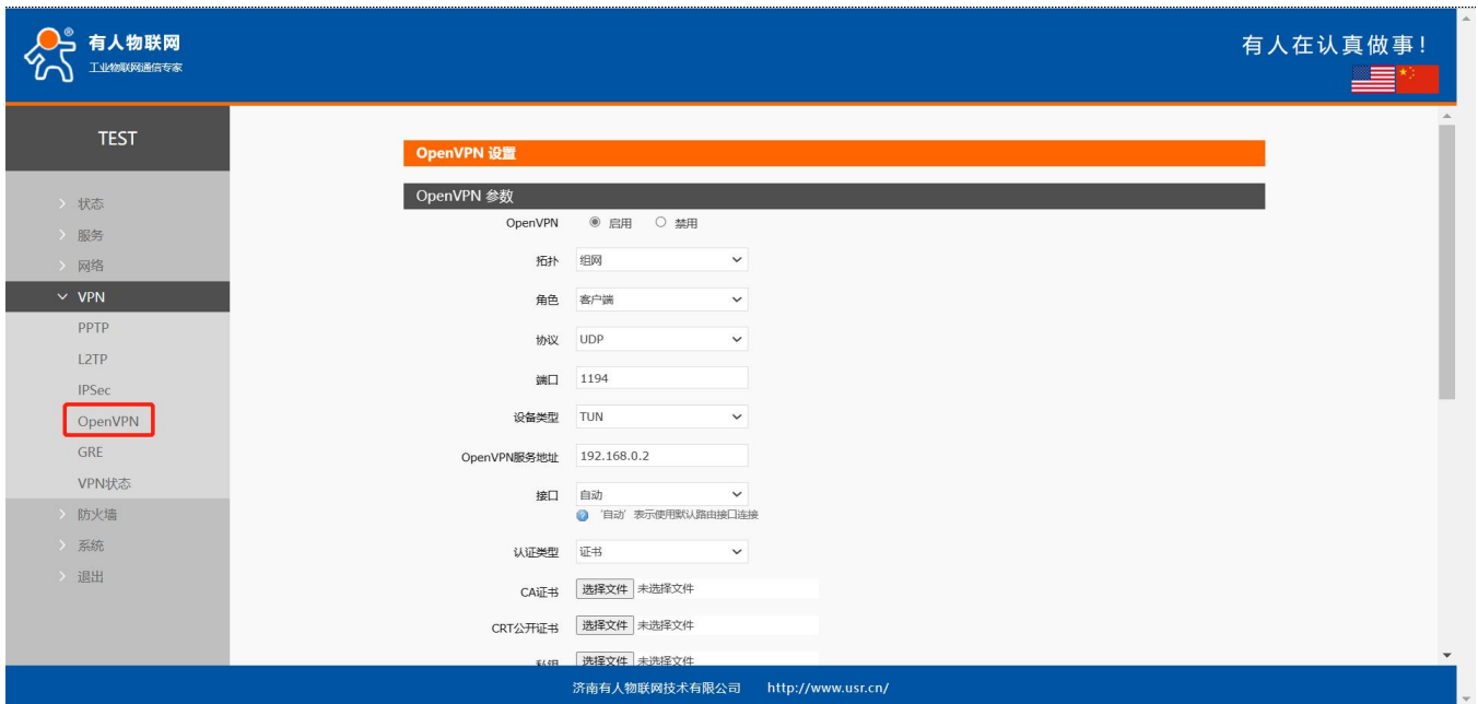
图 27 OpenVPN 启用设置界面
