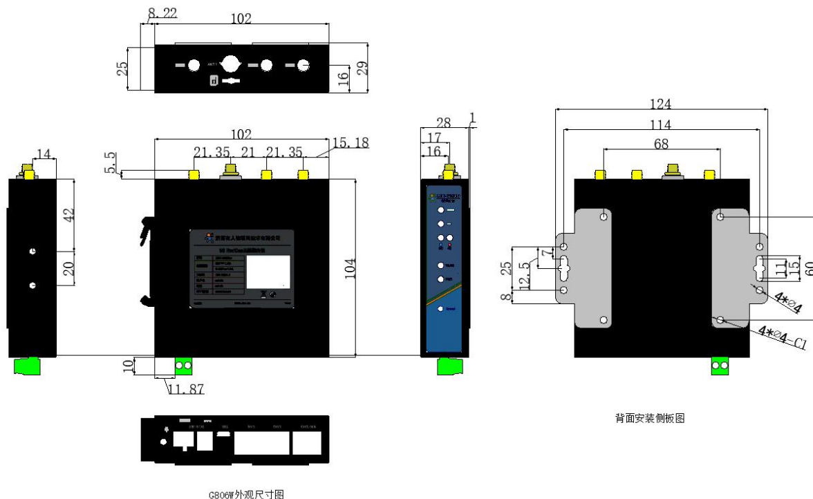
图 1 USR-G806R 尺寸图
