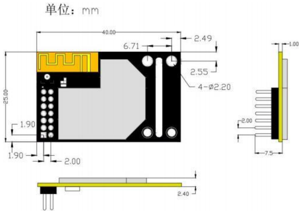
图 8 USR-WIFI232-A2 尺寸图
