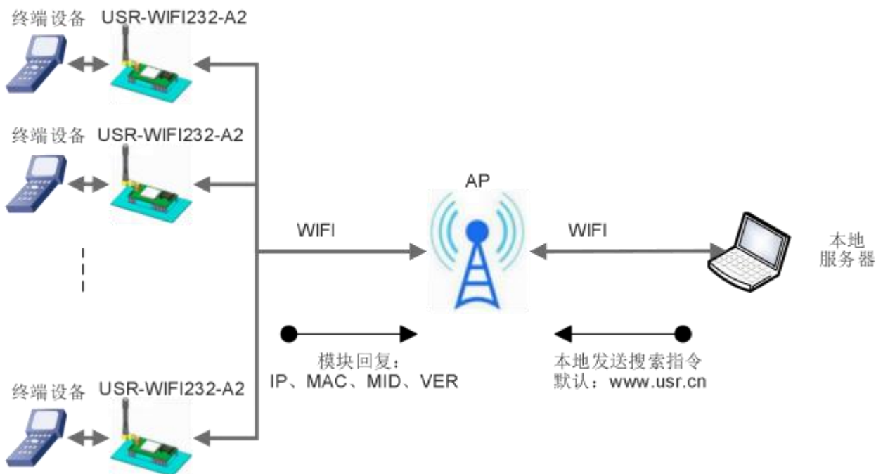
图 40 局域网搜索框图
