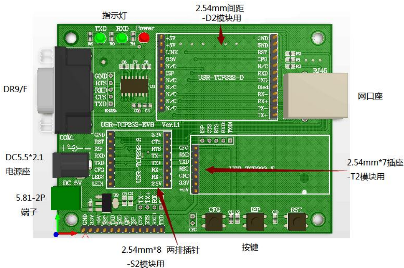
图 3 USR-TCP232-S2 模块评估板
