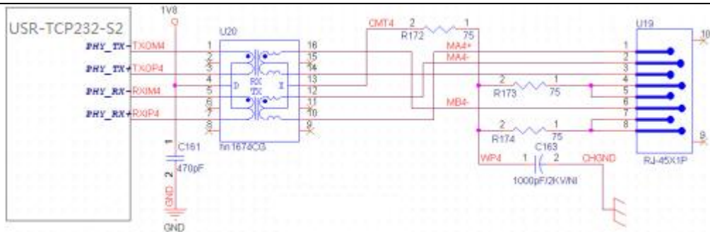
图 7 USR-TCP232-S2 以太网接口变压器接应用图
