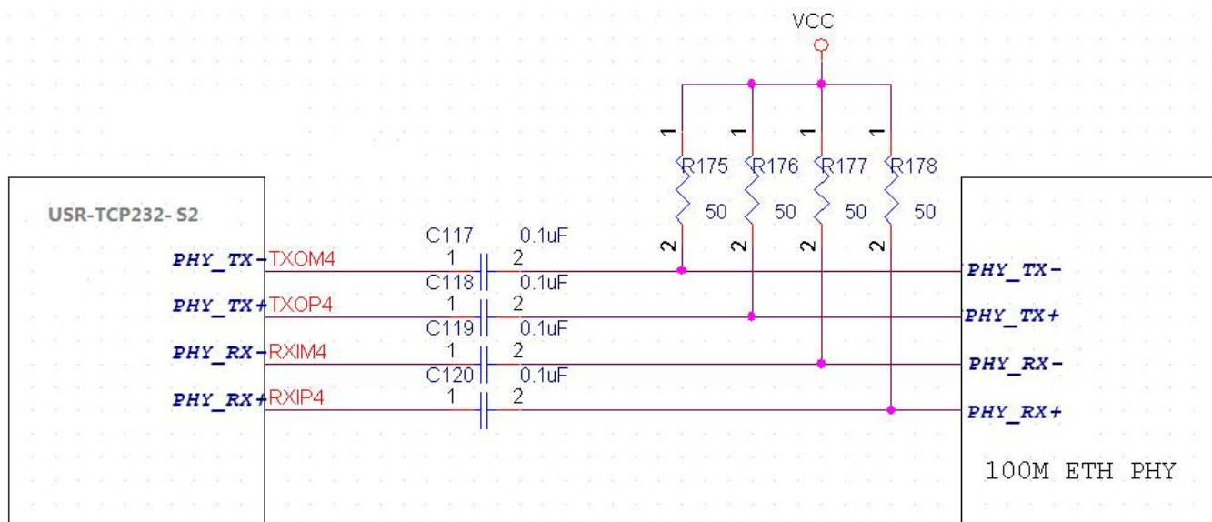
图 8 USR-TCP232-S2 以太网接口不带变压器接应用图
