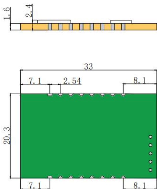
图 2 USR-TCP232-S2 尺寸图
