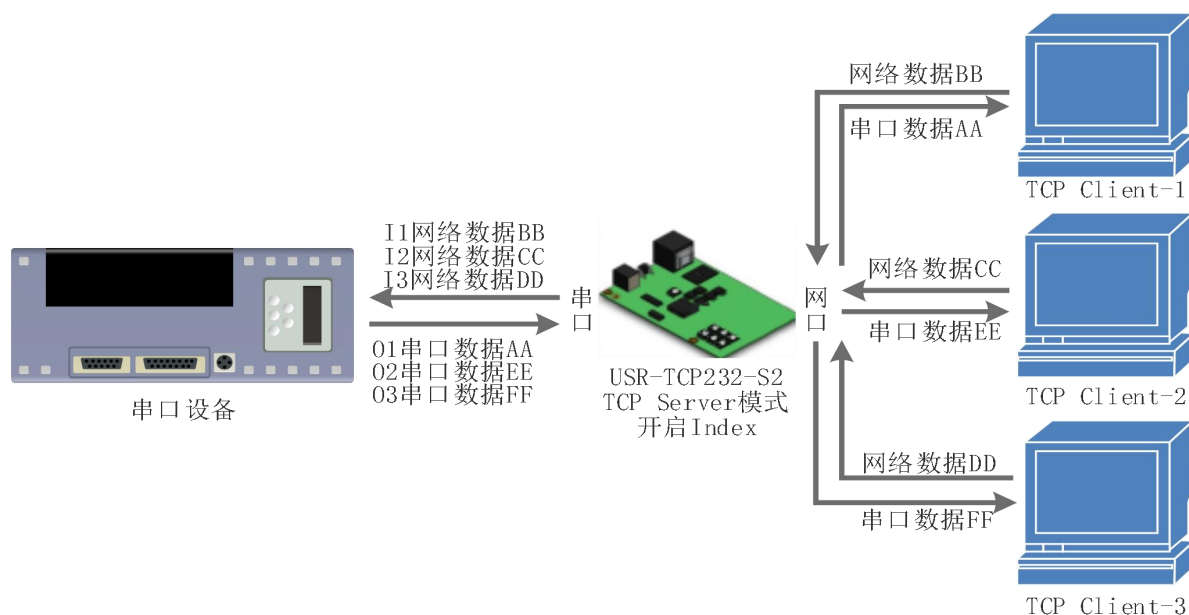
图 35. Index 功能示意图
