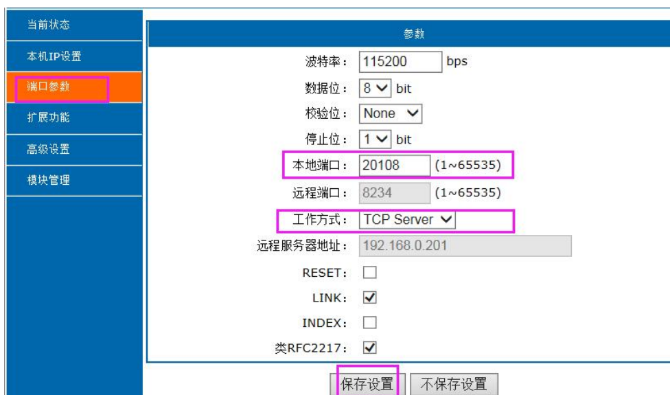
图 13. TCP Server 网页设置图
