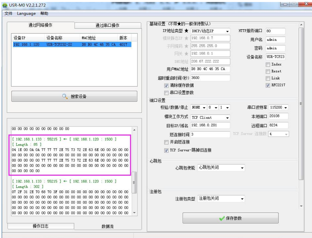
图 41. 抓取报文例如
