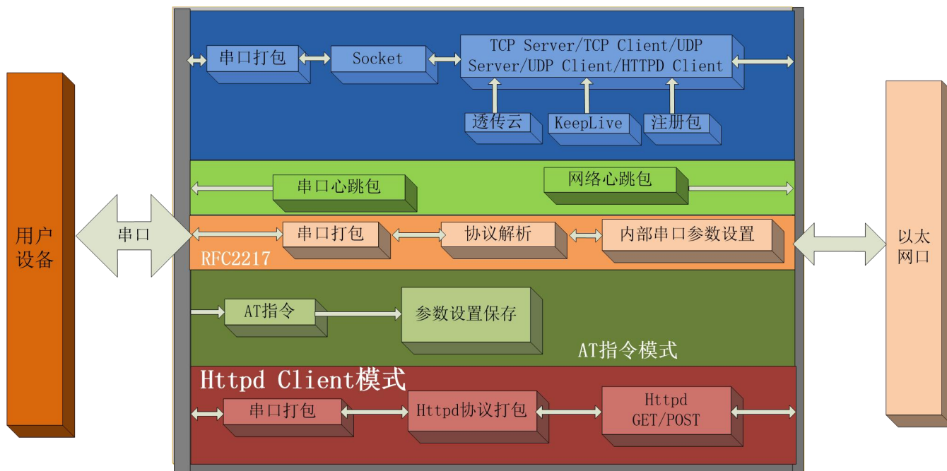
图 1. S2 功能框图
