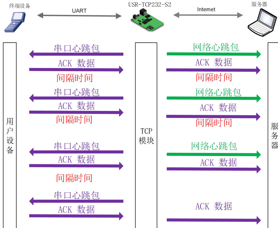
图 27. 心跳包功能示意图
