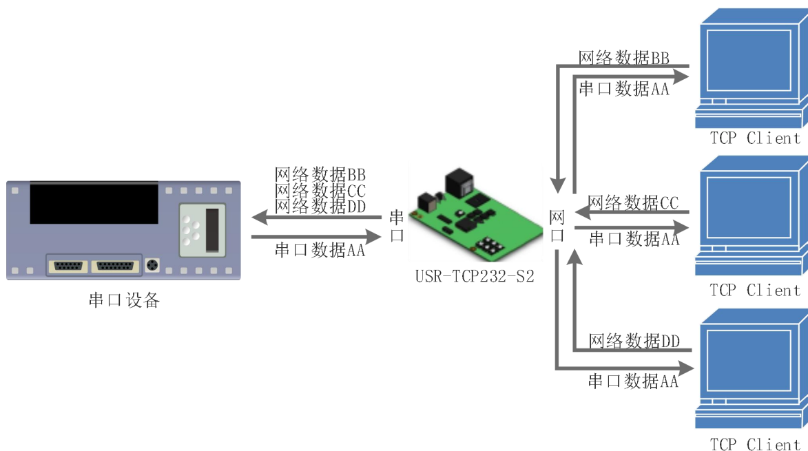
图 11. TCP Server 模式说明
