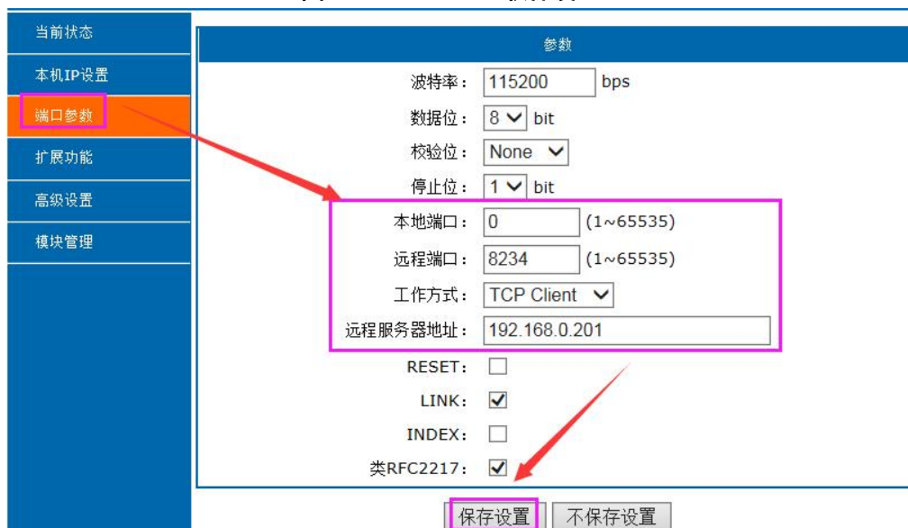
图 9. TCP Client 网页设置
