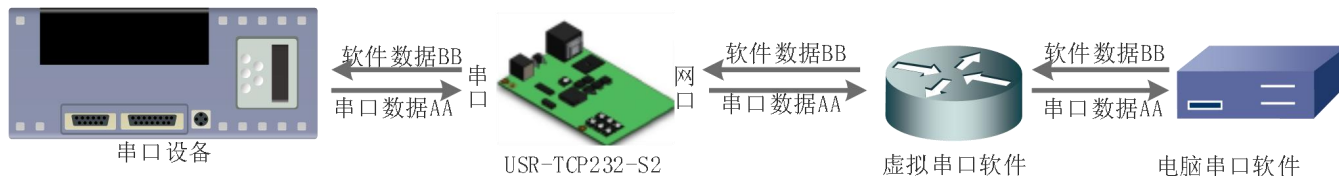
图 23. VCOM 应用介绍
