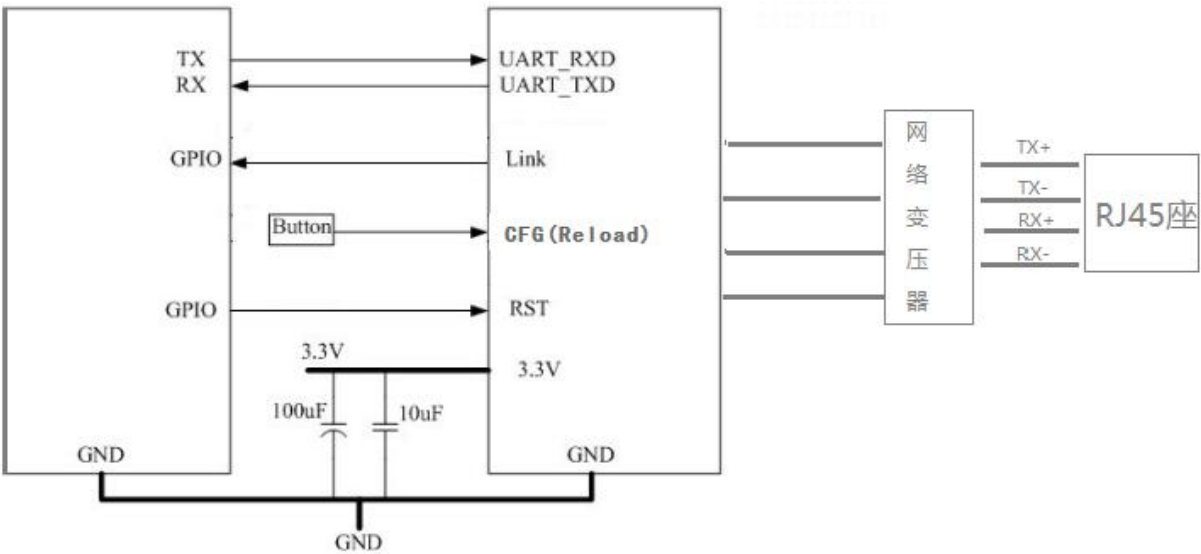
图 8. 硬件连接图
