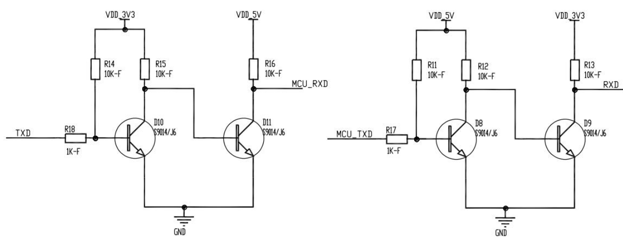
图 5. UART 电平转换参考设计
