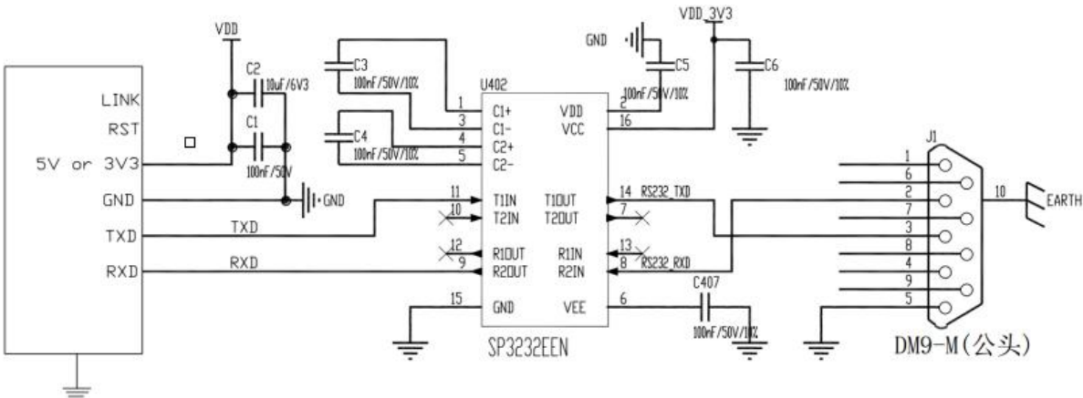
图 9. UART 接口参考设计
