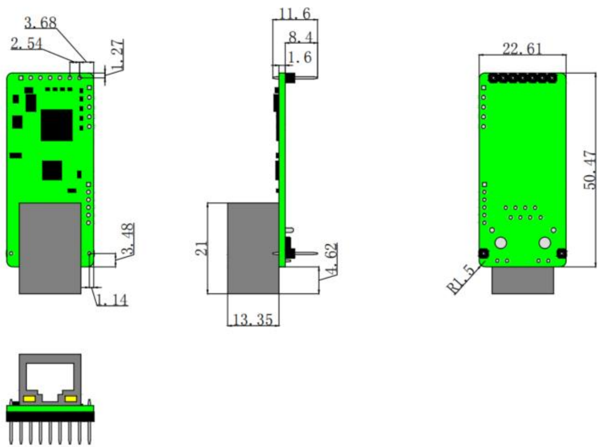
图 2. USR-TCP232-T1 尺寸图
