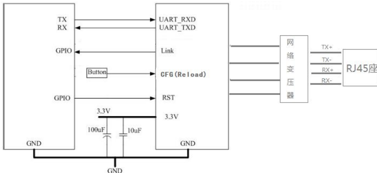
图 8. 硬件连接图
