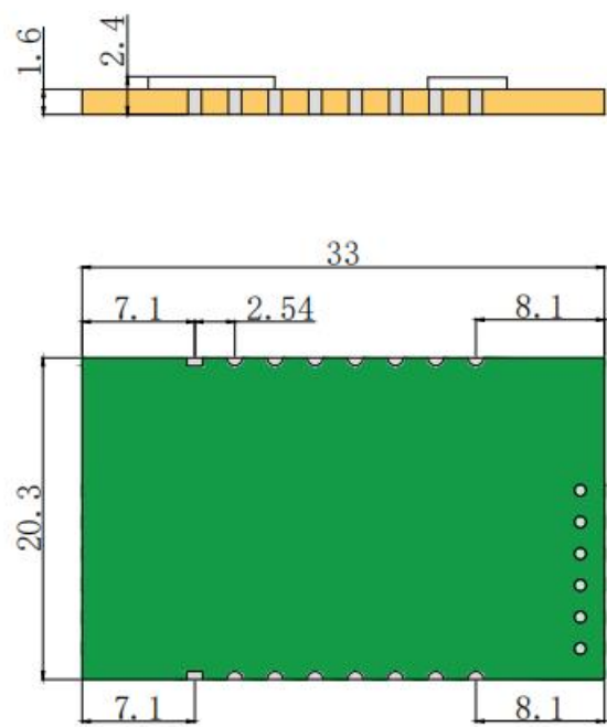
图 7. USR-TCP232-S1 产品尺寸图
