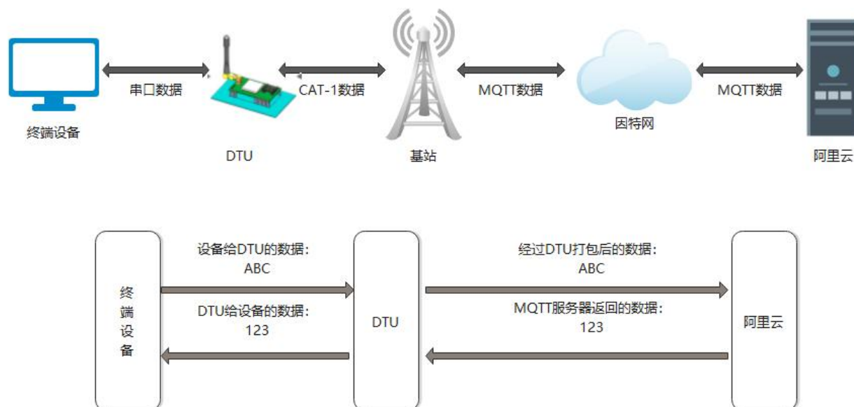
图 22. MQTT 模式
