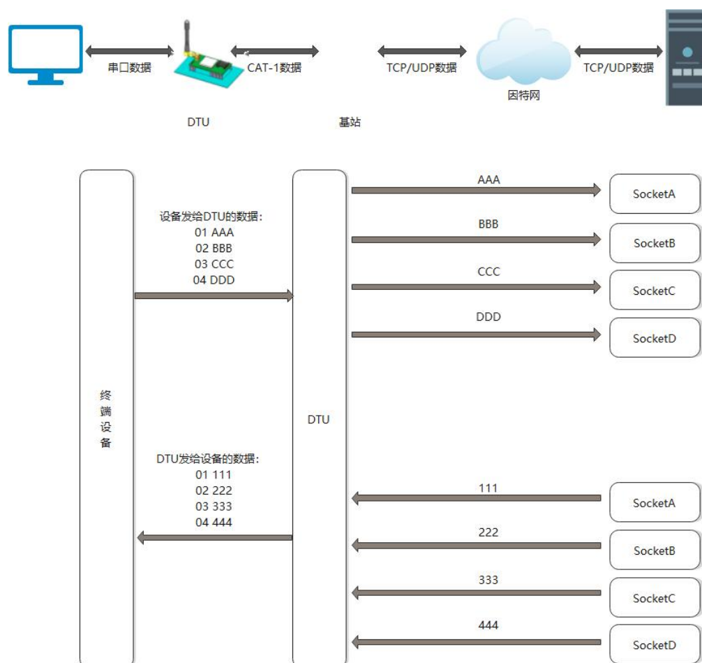
图 66. 套接字分发协议示意图
