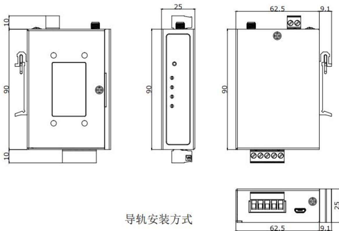
图 1. 导轨安装尺寸图
