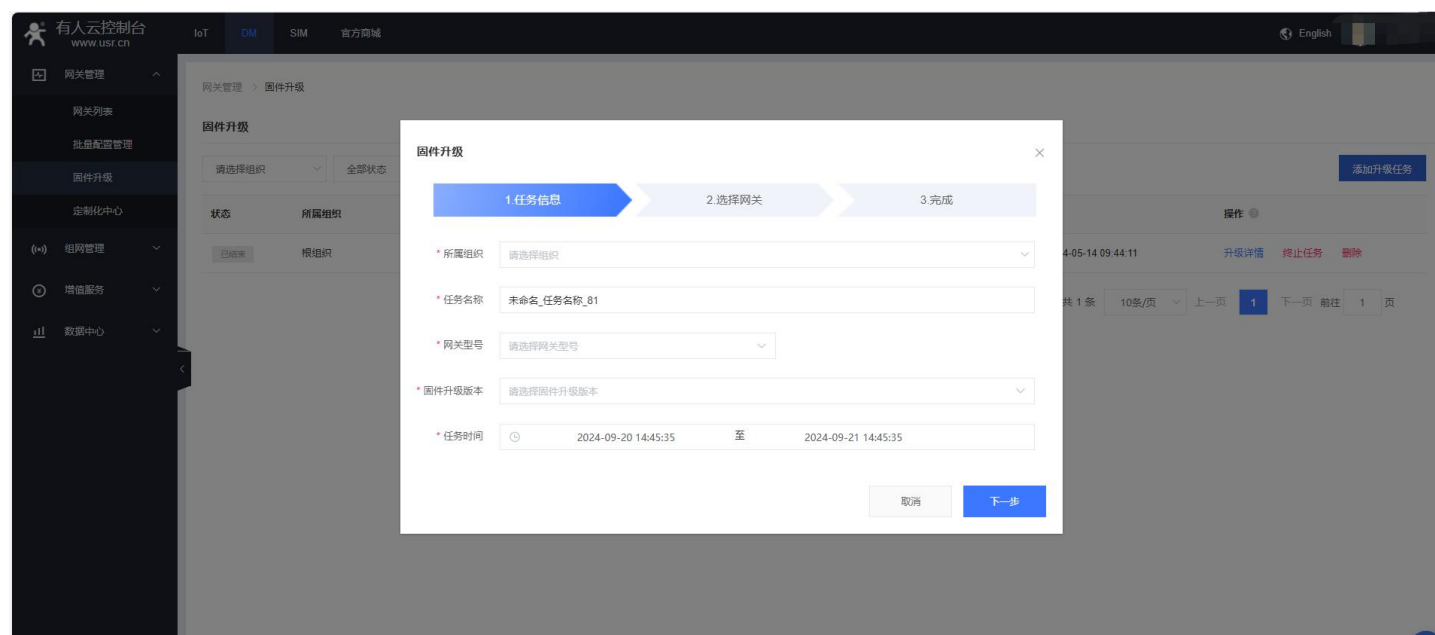
图 48. 固件升级
