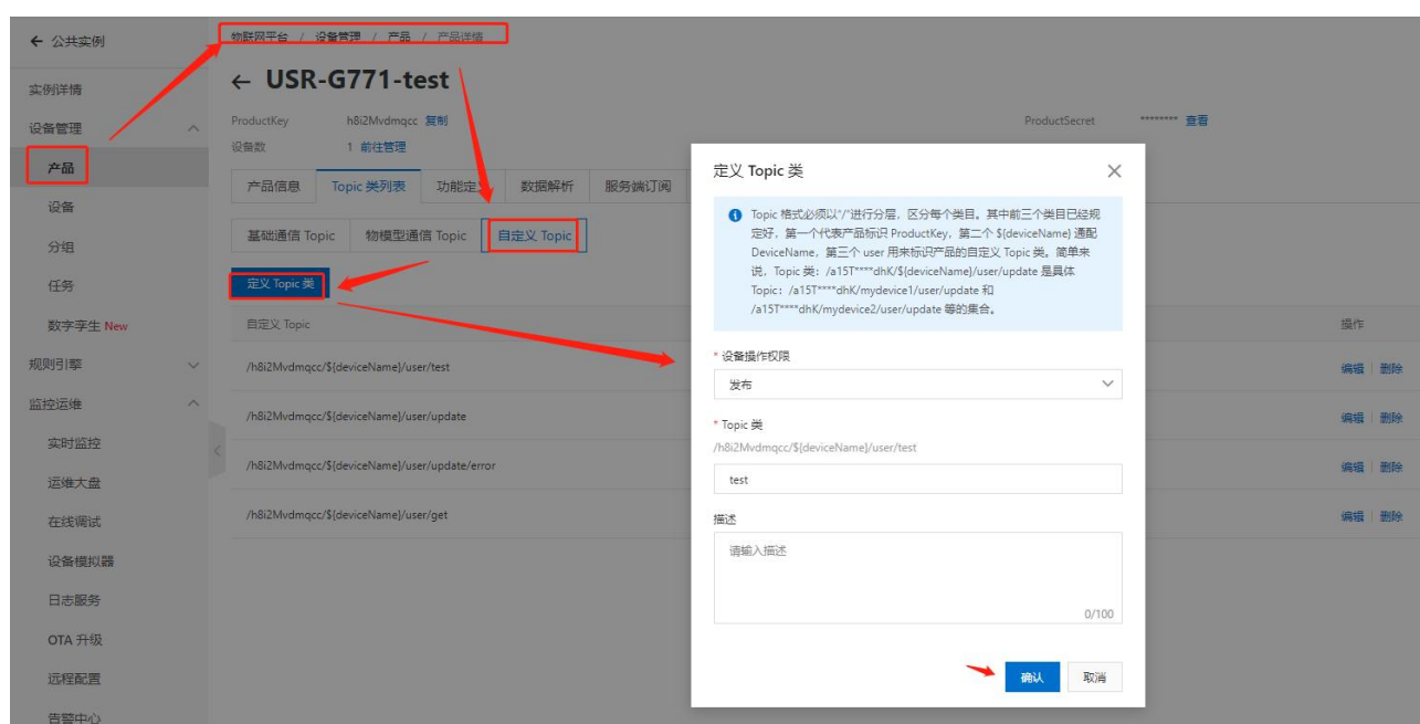
图 40. 自定义主题
