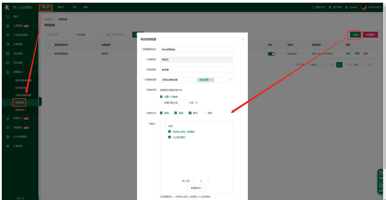
图 52. 报警配置
