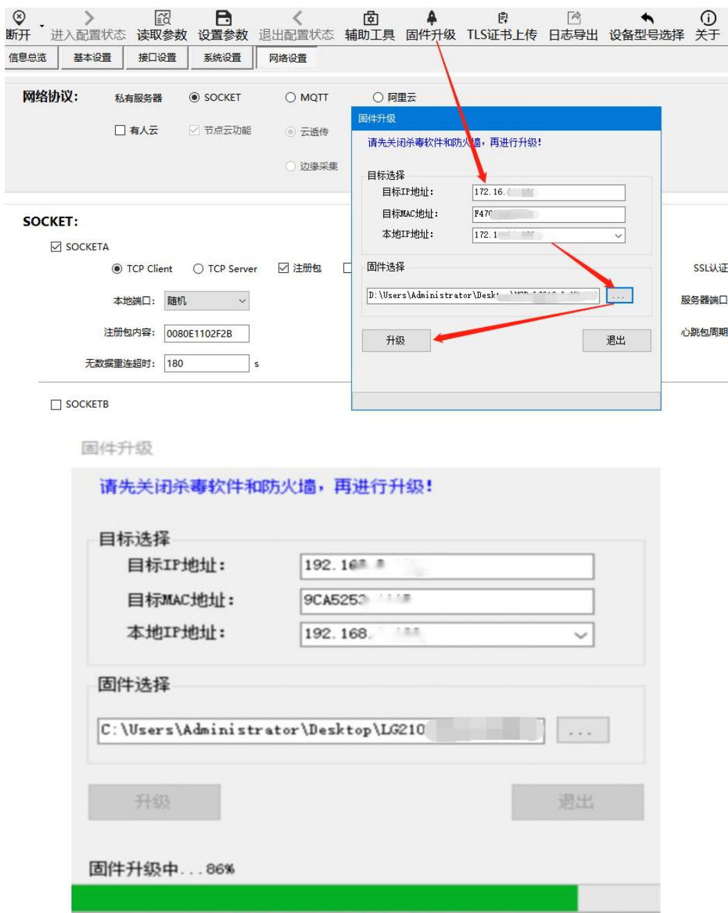
图 5-6 固件升级示意图
