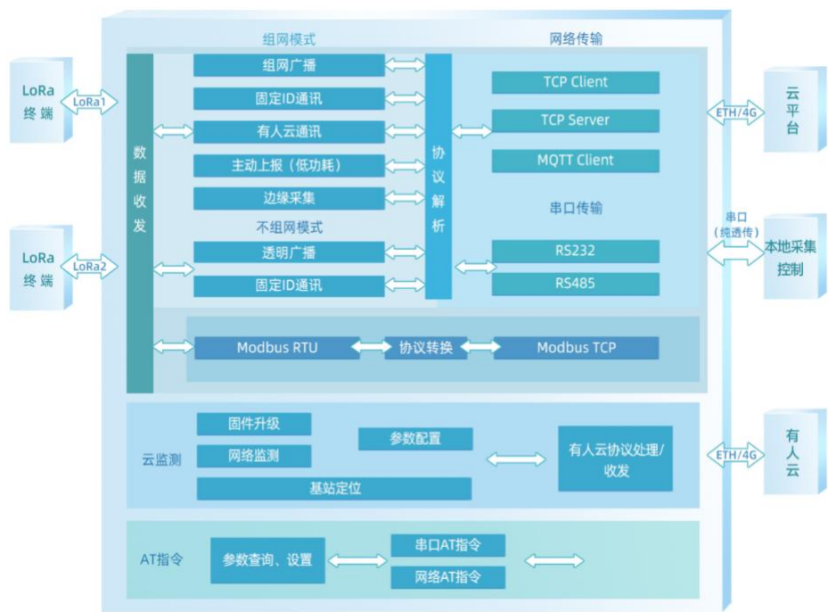
图 2-1 功能结构图
