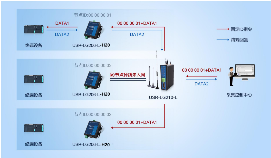
图 4-2 通信过程
