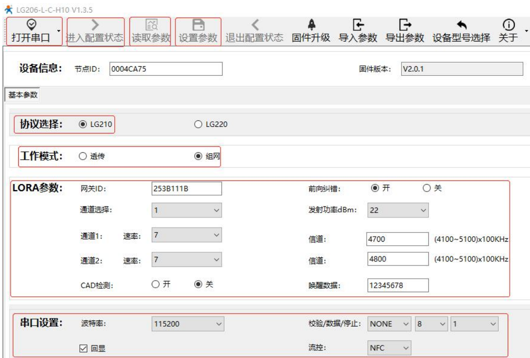
图 4-6 设置示例
