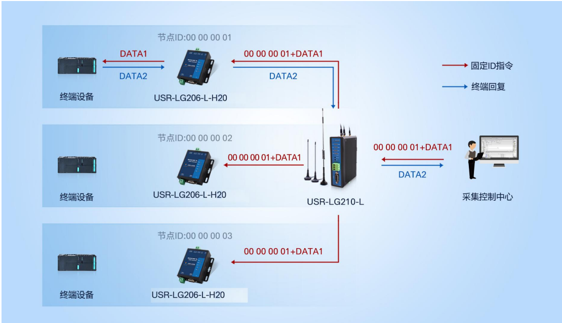
图 4-32 通信用程示意图
