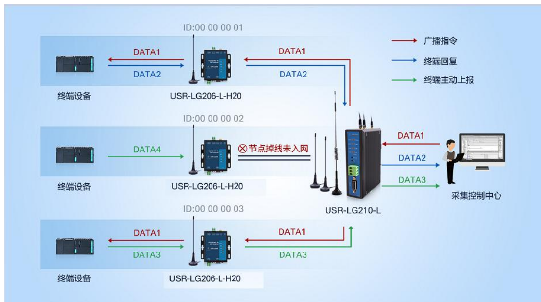
图 4-10 通信过程示意图
