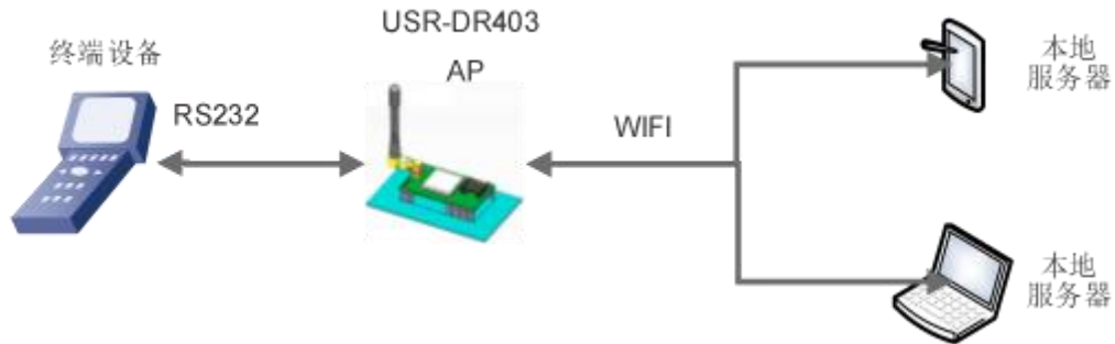
图 25 无线组网应用 (AP)
