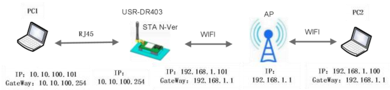
图 33 有线加无线组网应用 (路由)
