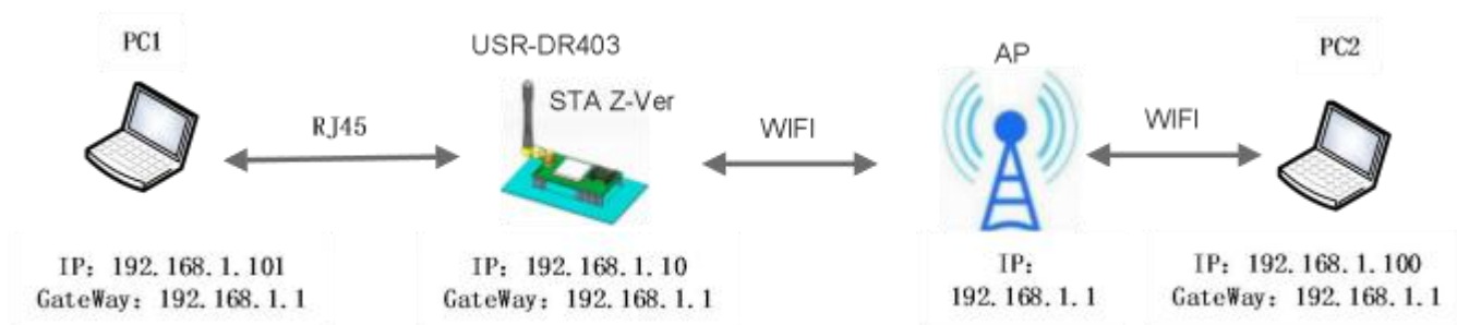
图 35 有线加无线组网应用（桥接）
