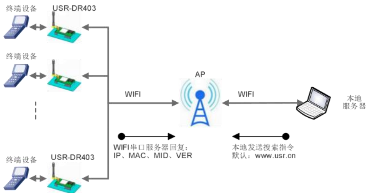
图 51 局域网搜索框图
