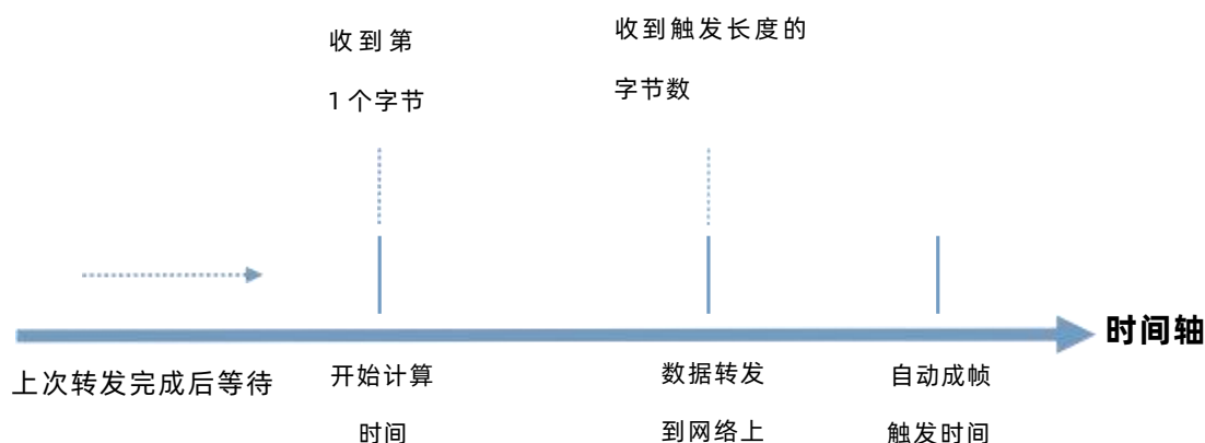
图 49 自动成帧触发帧长
