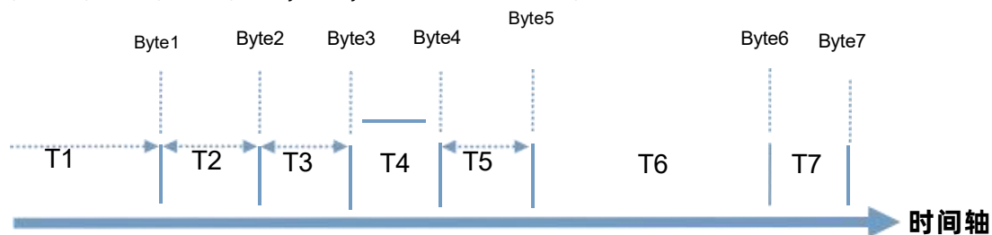
图 48 切换指令模式时序
