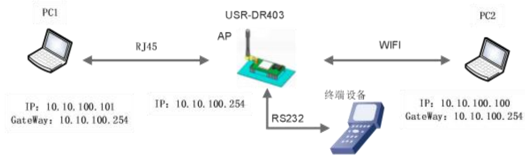
图 31 有线加无线的应用场景 (AP LAN)
