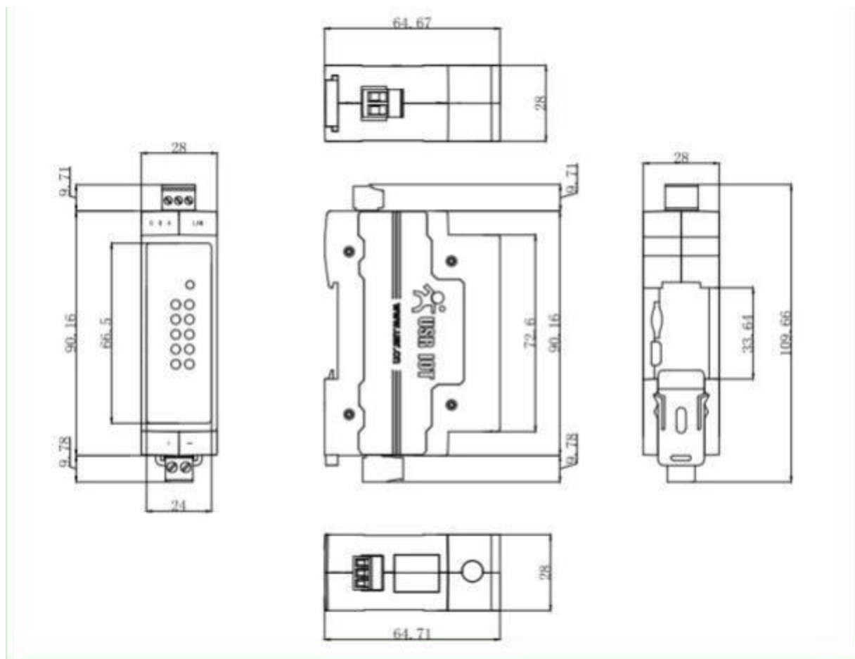
图 8 USR-DR403 外观尺寸图
