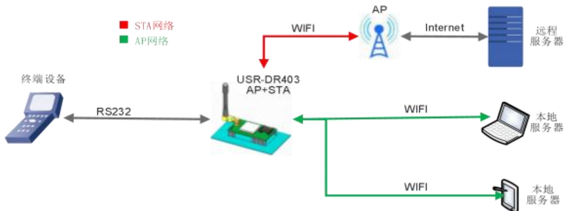
图 27 无线组网应用 ( AP+STA)
