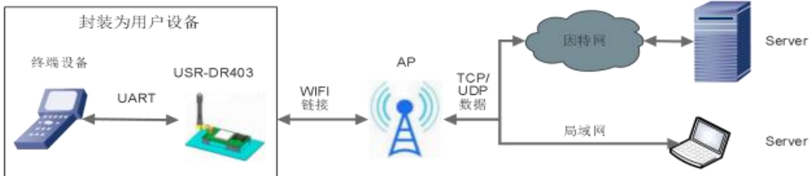
图 6 串口服务器基本功能
