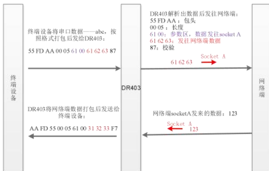
图 60 套接字分发框图
