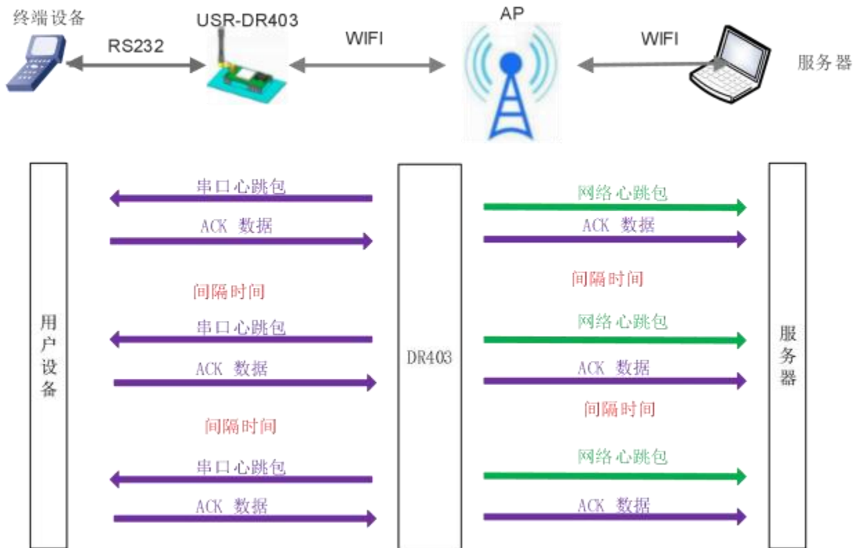
图 59 自定义心跳包功能框图
