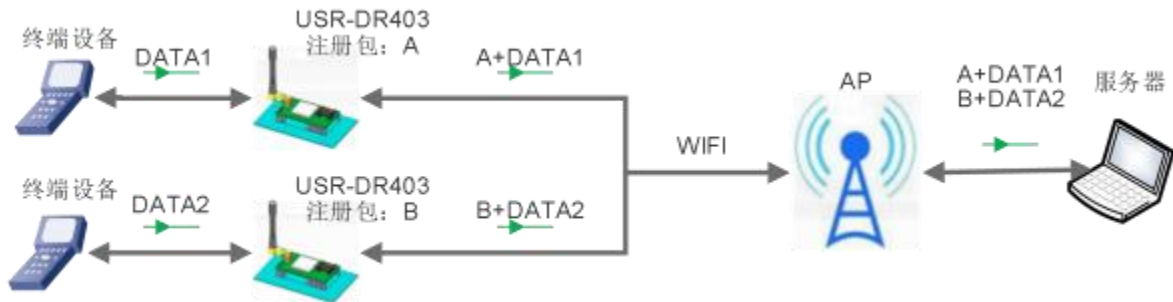
图 52 首次连接发送注册包框图
